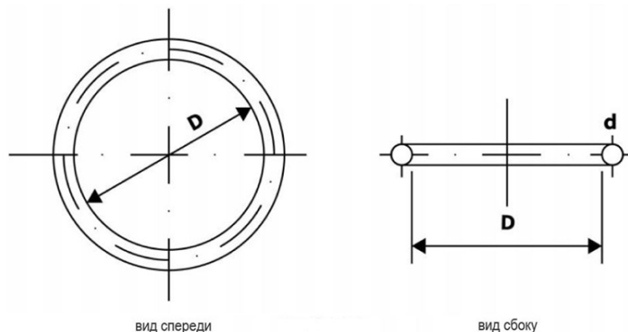
Типы уплотнительного кольца O-Ring
