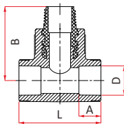
Тройник комбинированный HP
