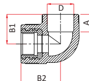
Угол 90° комбинированный BP
