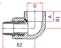
Угол 90° комбинированный HP
