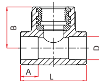
Тройник комбинированный BP
