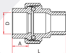
Муфта разъемная шестигранная НР типа "американка"
