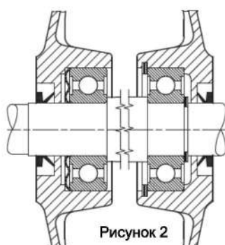
Схемы подшипников
