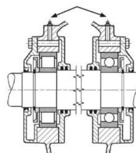
Схема подшипников Пресс-масленки
