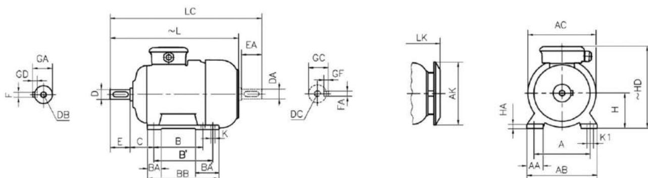
Размеры двигателей с креплением на ножках: схема крепления B3, B6, B7, B8, B15, V5, V6
