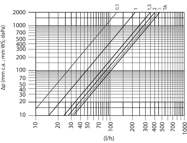
Графики пропускной способности узла R383 при двухтрубном подключении (байпас закрыт)
