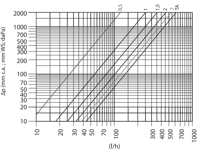
Графики пропускной способности узла R384 при двухтрубном подключении (байпас открыт)
