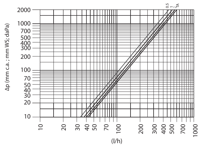
Графики пропускной способности узла R383 при однотрубном подключении
