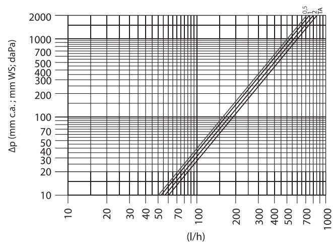
Графики пропускной способности узла R384 при однотрубном подключении (байпас открыт)
