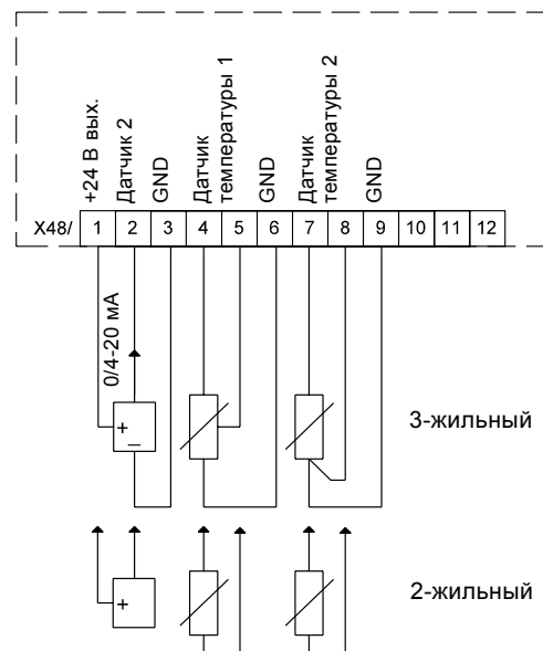
Fig. 55 Схема электрических соединений, МСВ 114
