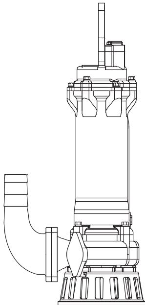
5-сур. Сақиналы негіздегі тасымалданатын қондырғы
