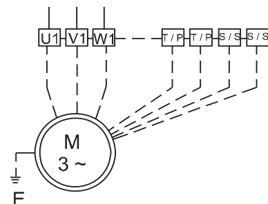
6-сур. Электрлік қосылыстар схемалары, тікелей қосу
