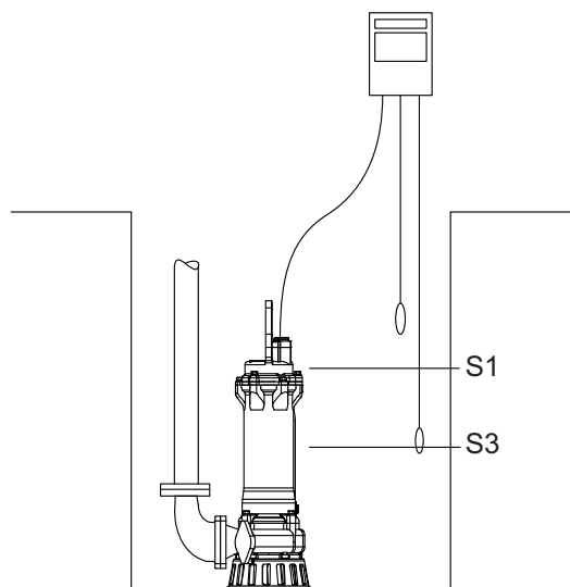
Рис. 10 Уровень жидкости
