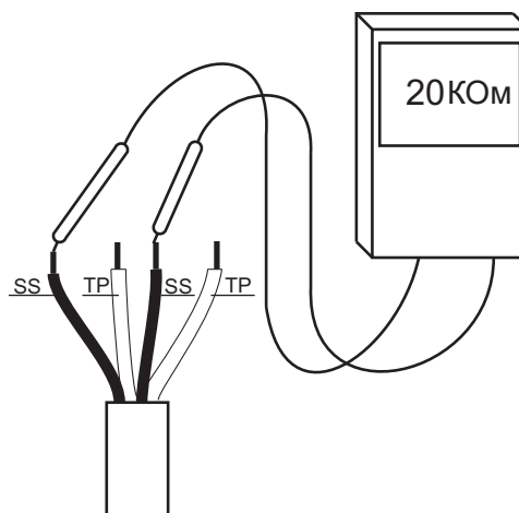
Рис. 13 Проверка сопротивления
