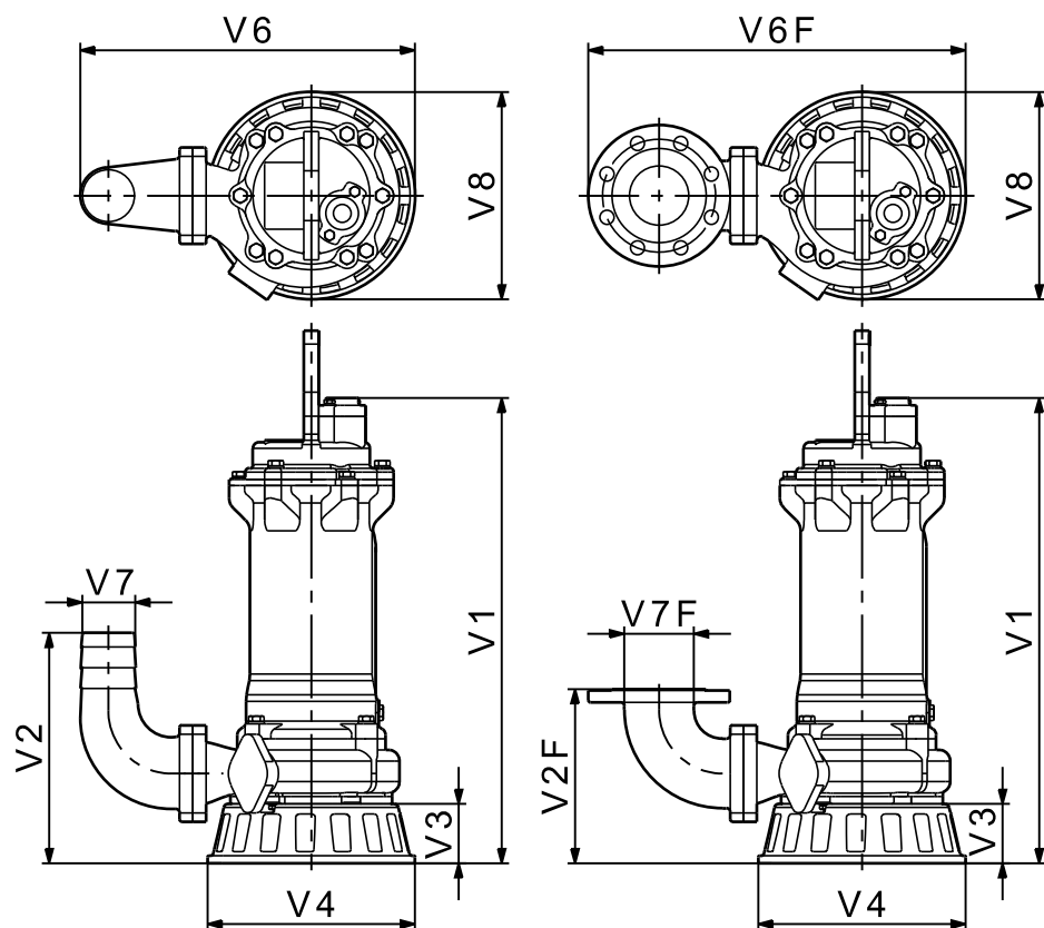
Рис. 15 Размеры при установке насоса на кольцевом основании
