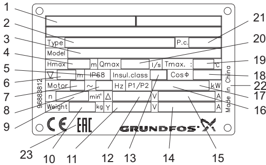
Рис. 3 Фирменная табличка
