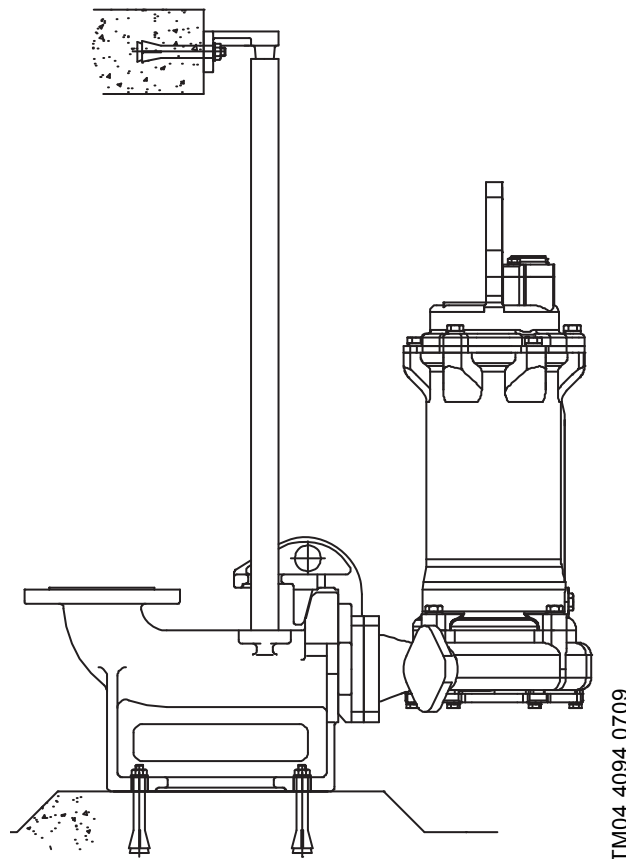
Рис. 4 Погружной насос на автоматической трубной муфте
