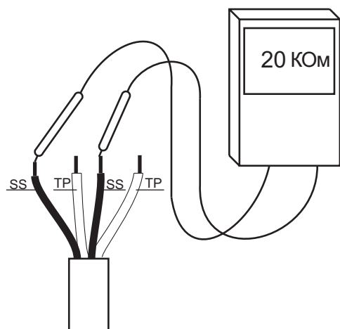
Рис. 11 Проверка сопротивления
