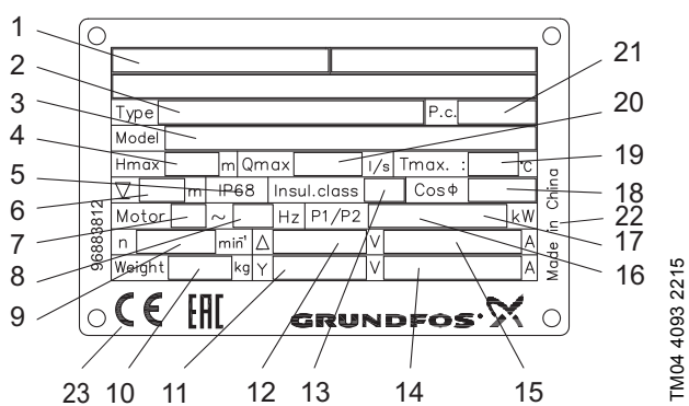
Рис. 2 Фирменная табличка
