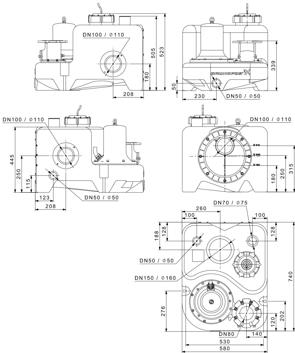
Рис. 34 Габаритные размеры
