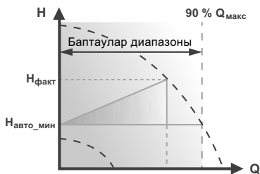
32-сур. FLOW_{ADAPT}
