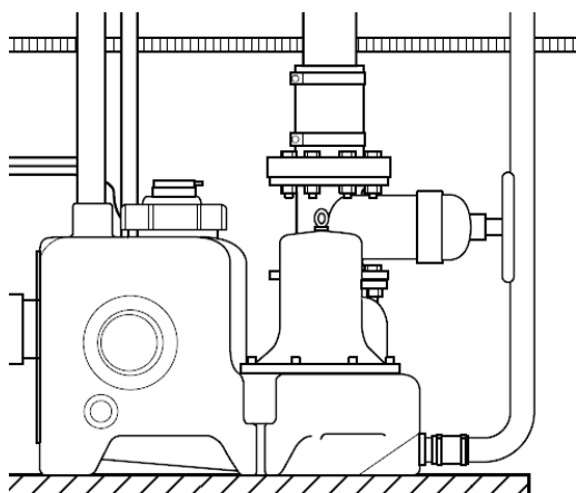
Рис. 19 Здвижка на обратном клапане
