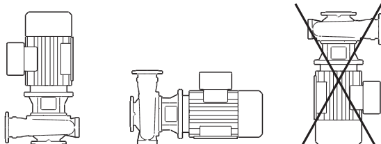
Рис. 9 Варианты монтажа
