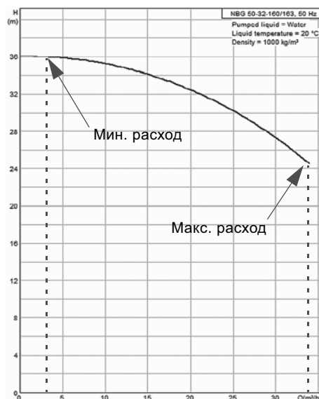
Рис. 24 Пример с указанием минимального и максимального расхода
