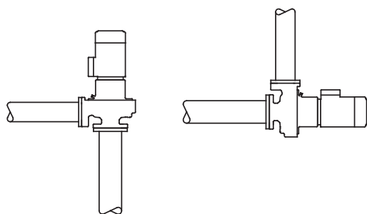
Рис. 17 Прямое соединение насоса с трубопроводом
