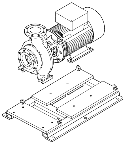
14-сур. Құюға арналған саңылауымен тақта-негіз
