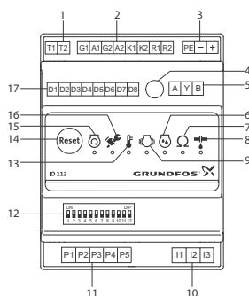
Рис. 15 Модуль IO 113
