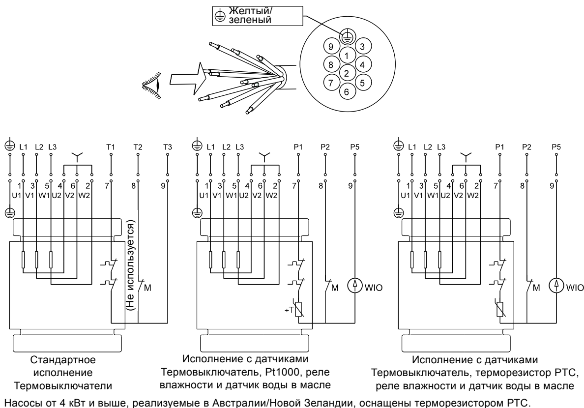
Рис. 10 Схема электрических соединений для 10-жильного кабеля, соединение звездой (Y)
