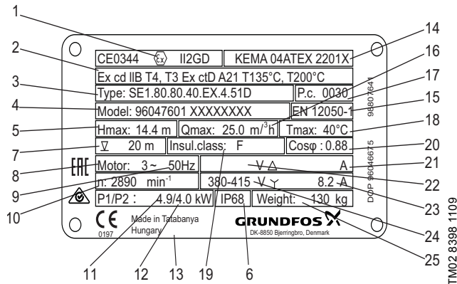
Рис. 2 Фирменная табличка
