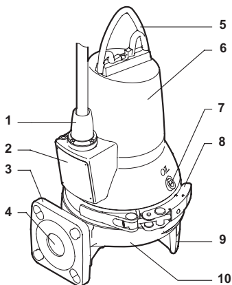
1-сүр. SEG соркысмасы
