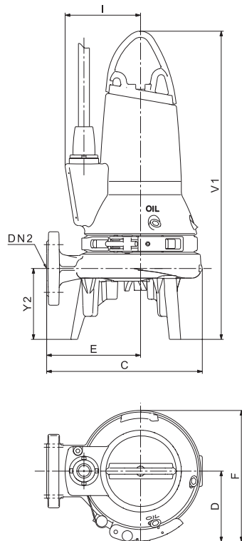
Рис. 18 Переносная установка с удлинёнными опорными ножками
