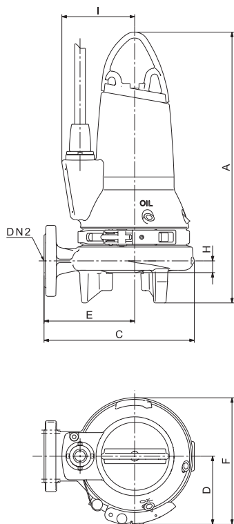
Рис. 17 Переносная установка
