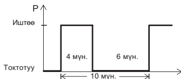
10-сүр. S3 иш режимі
