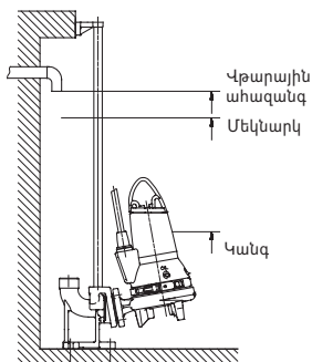
Նկար 7 Պոմպի գործարկման և շարժականգի մակարդակները
