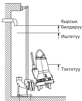
7-сүр. Коё берүүнүн деңгээлдери жана соркысманын токтошу
