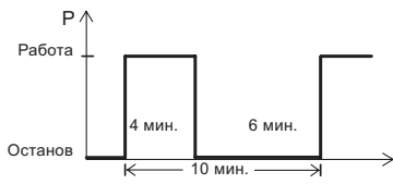
Рис. 10 Режим работы S3
