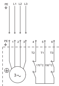
6-сур. Үш фазалы электрлі қозғалтқыштармен сорғылардың қосылыстар схемасы
