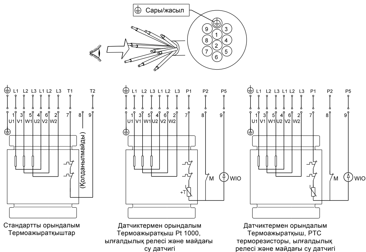
10-сур. 10-тармақты кабельге арналған электрлік жалғанымдар сызбасы, «жұлдыз-үшбұрыш» жалғаным (Y/D)
