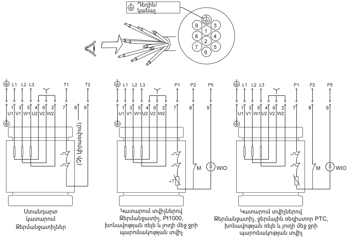
Նկար 11 10-ջիղանի մալուխի համար էլեկտրական միացումների սխեմա, միացում ,աստղե (Y)
