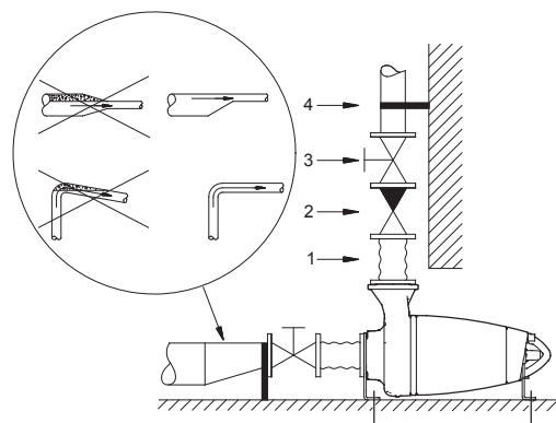
Сүр. 6 Туурасынан абалда тирөөчтөргө орнотулган кургак орнотуу
