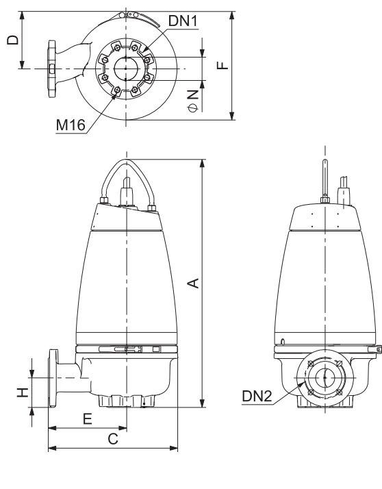
Рис. 29 Насос SEV без принадлежностей
