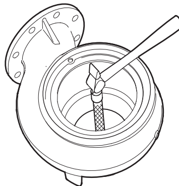
26-сур. Тығыздағыш шығыршықты құрастыру
