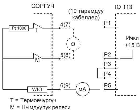
Сүр. 16 Pt1000 менен SE1, SEV соркысмалар
