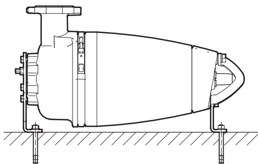
Նկար 8 Հենակների վրա չոր տեղադրում՝ հորիզոնական դիրքում
