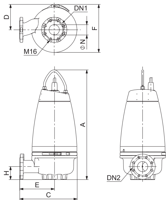
Рис. 30 Насос SEV без принадлежностей
