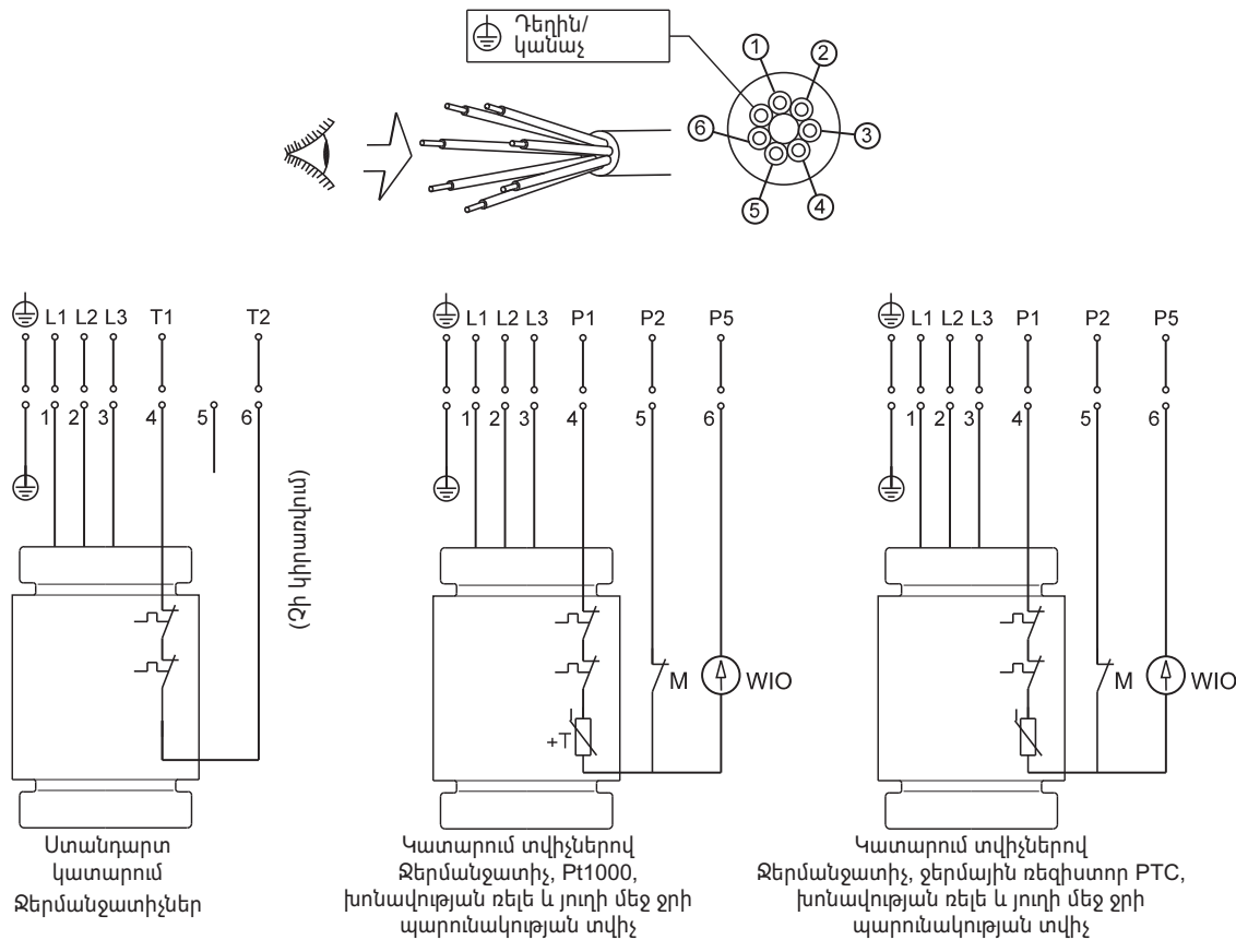
Նկար 9 7-ջիղանի մալուխի համար էլեկտրական միացումների սխեմաներ, ուղղակի մեկնարկ
