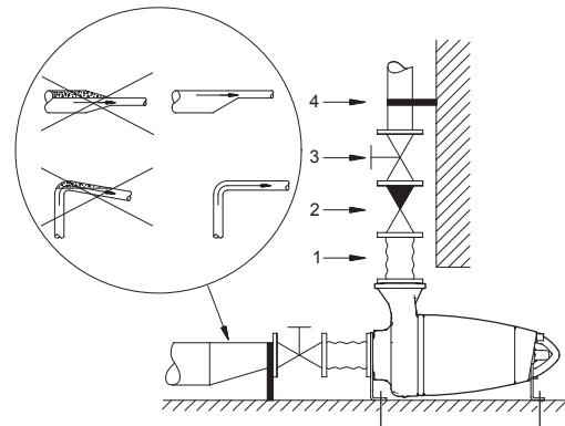
Նկար 6 Հենակների վրա չոր տեղադրում՝ հորիզոնական դիրքում
