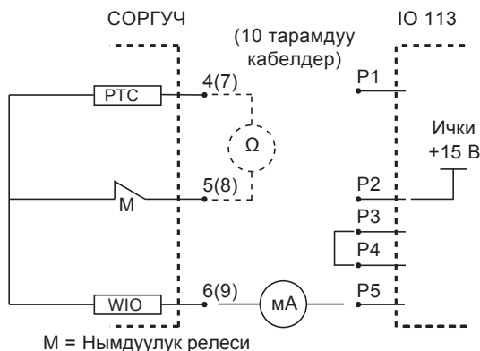
Сүр. 17 PTC билдиргичи менен SE1, SEV соркысмалар
