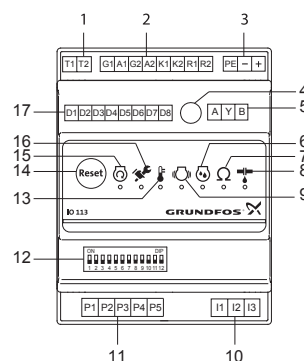
Сүр. 15 IO 113 модулу
