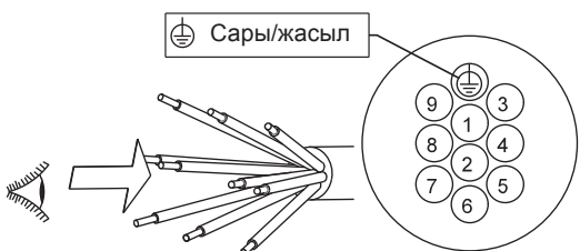
11-сур. 10-тармақты кабельге арналған электрлік жалғанымдар сызбасы, «жұлдыз» жалғанымы (Y)
