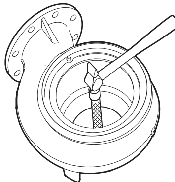
Сүр. 26 Тыгыздооч жээкти куруу
