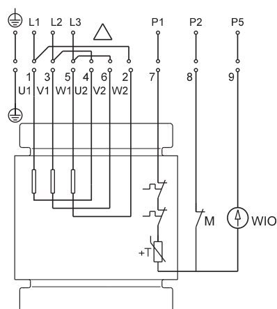
Датчиктермен орындалым Термоажыратқыш Pt 1000, ылғалдылық релесі және майдағы су датчигі
