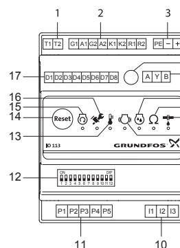
Рис. 15 Модуль IO 113
