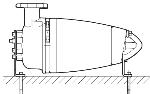
8-сур. Тіреулерде көлденең күйіндегі құрғақ орнатылым
