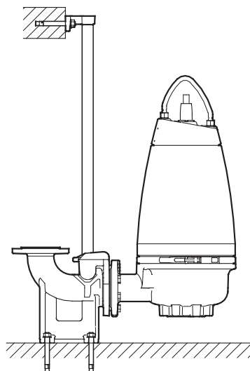
Сүр. 4 Автоматтык түтүк муфтага орнотулган чумкоо орнотуусу
