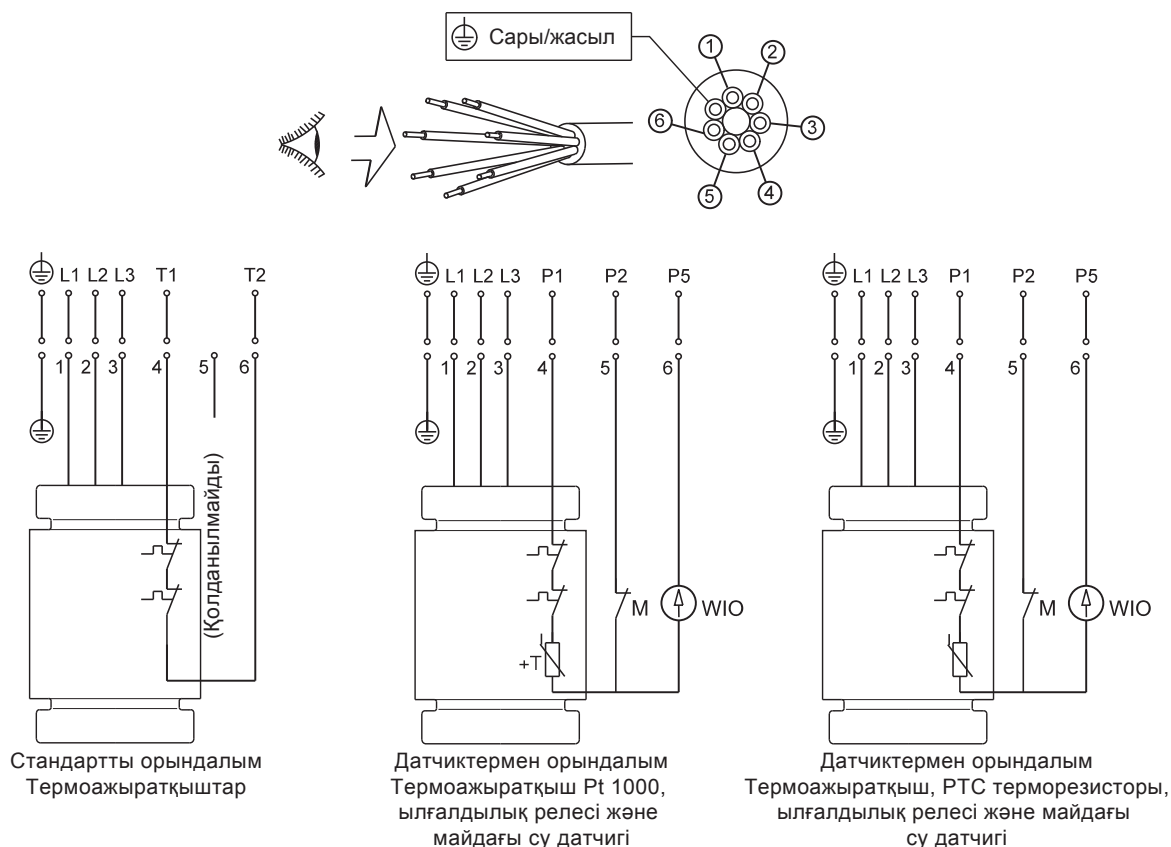
9-сур. 7-тармақты кабельге арналған электрлік жалғанымдар сызбасы, тікелей іске қосу
