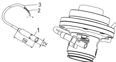
Сүр. 14 WIO билдиргичи
