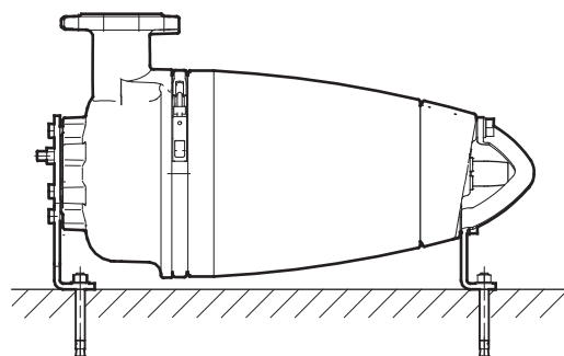
Сүр. 8 Туурасынан абалда тирөөчөргө орнотулган кургак орнотуу
