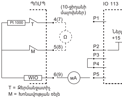
Նկար 16 SE1, SEV պոմպեր՝ Pt1000-ով
