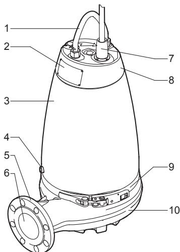
Նկար 1 Պոմպ SE
