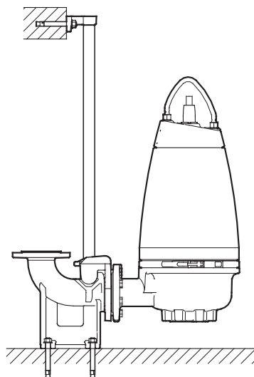
4-сур. Автоматты құбырлық жалғастырғыштағы батырма типінің құрастырылуы
