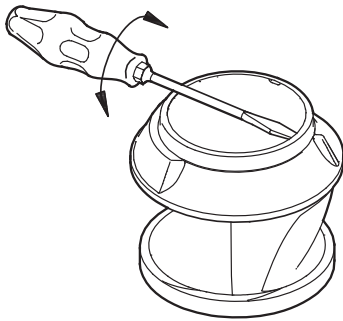
Նկար 25 Անցքի խցուկի օղակի ապամոնտաժում
