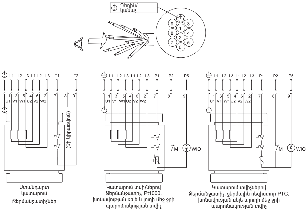
Նկար 10 10-ջիղանի մալուխի համար էլեկտրական միացումների սխեմաներ, միացում ,աստղ-եռանկյունի (Y/D)
