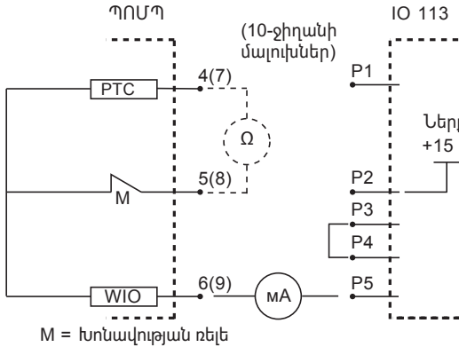
Նկար 17 SE1, SEV պոմպեր՝ PTC տվիչով
