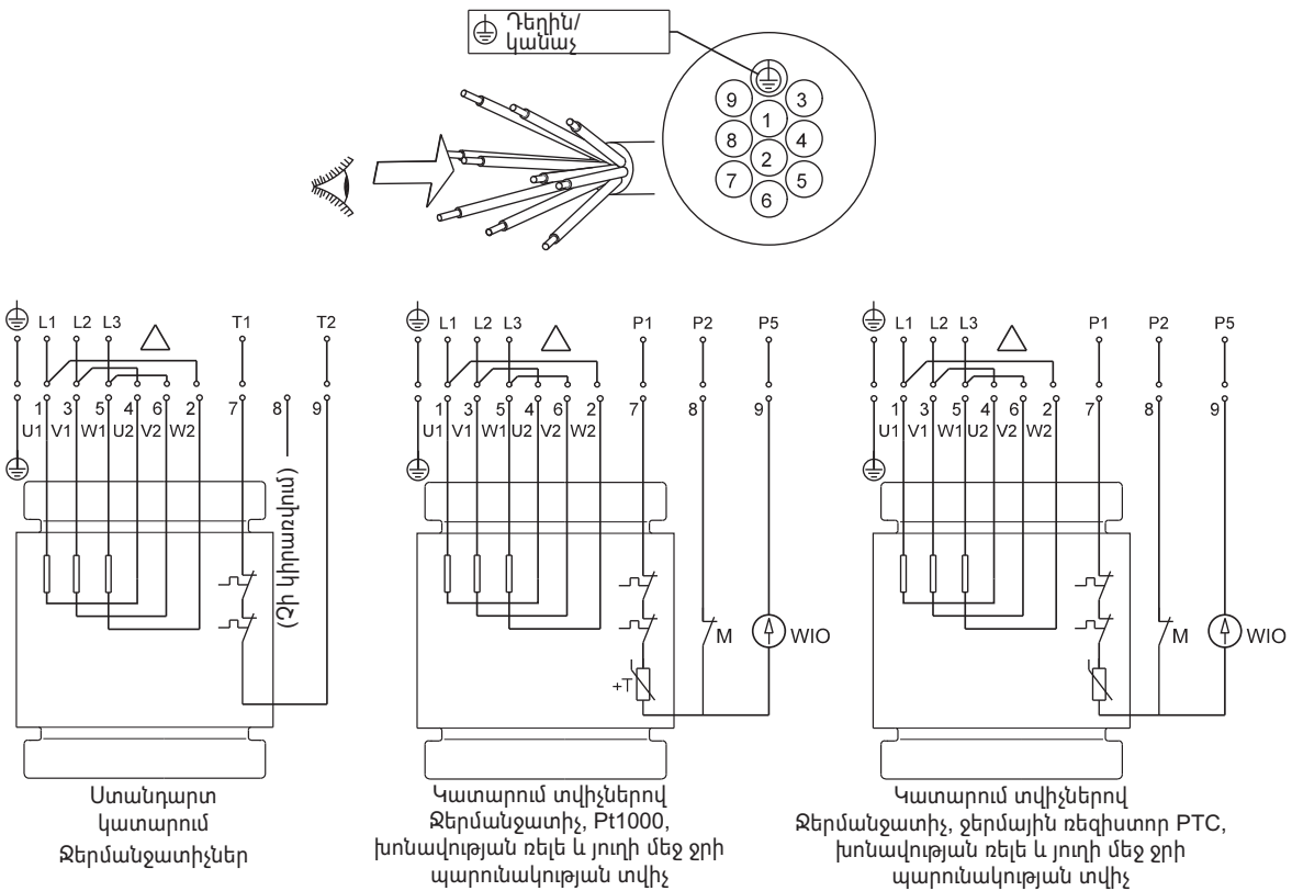
Նկար 12 10-ջիղանի մալուխի համար էլեկտրական միացումների սխեմա, միացում ,եռանկյունիե (D)
