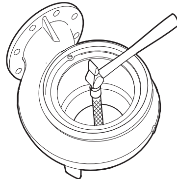
Նկար 26 խցուկային օղակի տեղադրում
