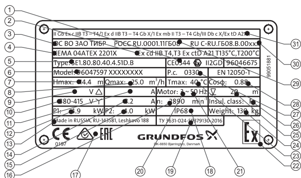
3-сур. Ресейде жасалған сорғыларға арналған фирмалық тақташа
