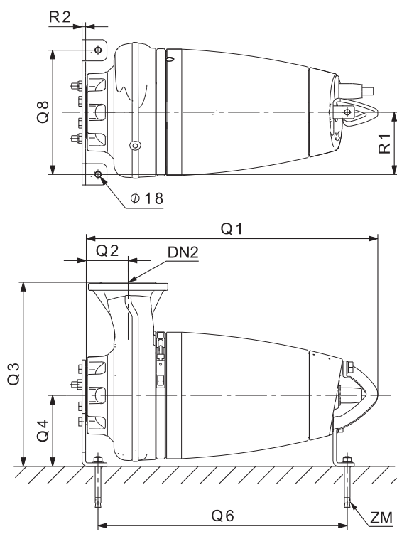
Рис. 35 SE1 Сухая горизонтальная установка
