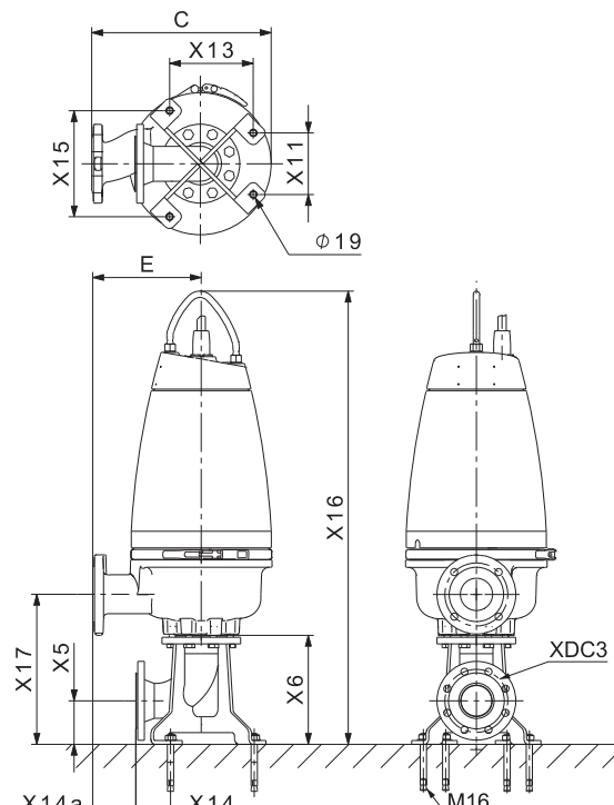
Рис. 44 Сухая установка насоса SEV в вертикальном положении
