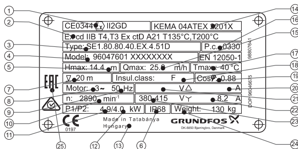
Рис. 2 Фирменная табличка
