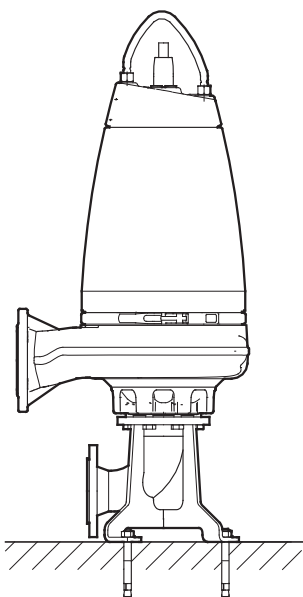
Նկար 7 Հիմքերի վրա չոր տեղադրում՝ ուղղահայաց դիրքում
