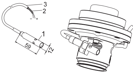
Նկար 14 WIO տվիչ
