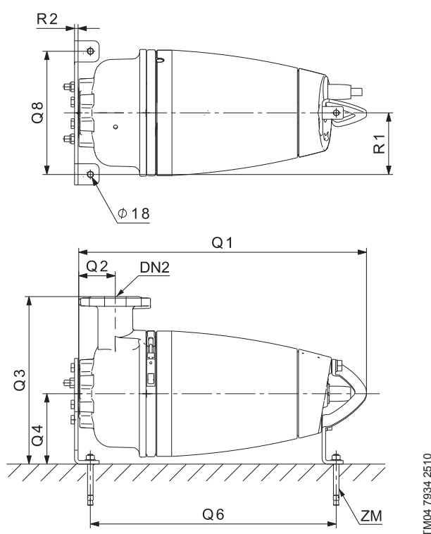
Рис. 36 SEV Сухая горизонтальная установка
