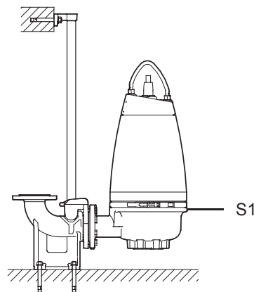
Նկար 20 Ավտոմատ խողովակային կցորդիչի վրա ընկղմվող տեղադրման տարբերակ
