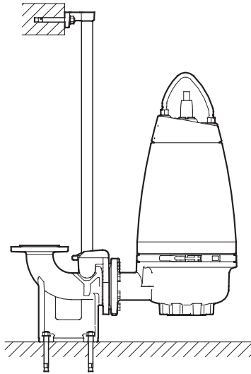
Նկար 4 Ավտոմատ խողովակային կցորդիչի վրա ընկղմվող տեղադրման տարբերակ
