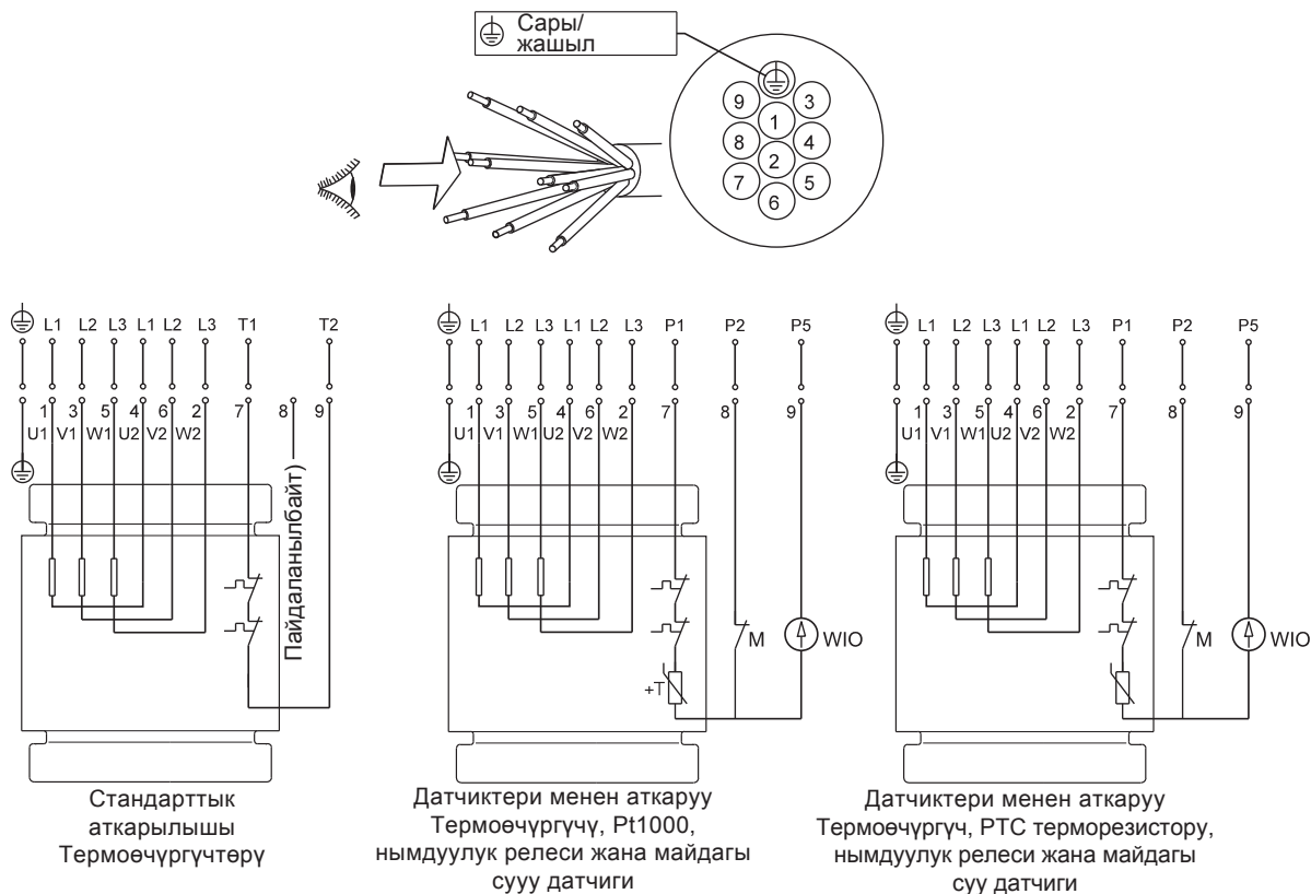
Сүр. 10 10-катмарлуу кабели үчүн электр туташуулардын түзмөктөрү, "жылдыз-үч бурчтук" туташуу (Y/D)
