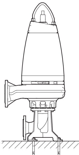
7-сур. Негізде тік күйіндегі құрғақ орнатылым
