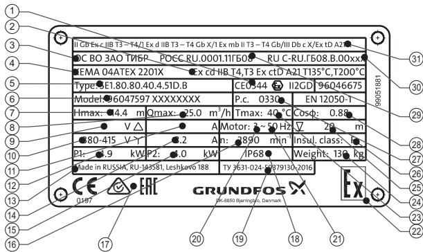
Նկար 3 Ֆիրմային վահանակներ Ռուսաստանում արտադրված պոմպերի համար
