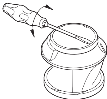
25-сур. Жарықтық тығыздағыш шығыршығын бөлшектеу
