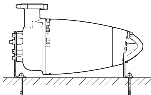
Рис. 8 Сухая установка на опорах в горизонтальном положении
