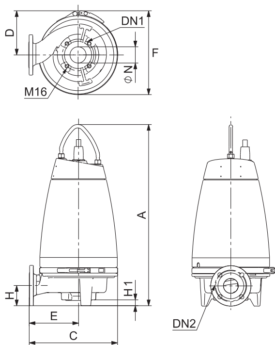
Рис. 27 Насос SE1 без принадлежностей
