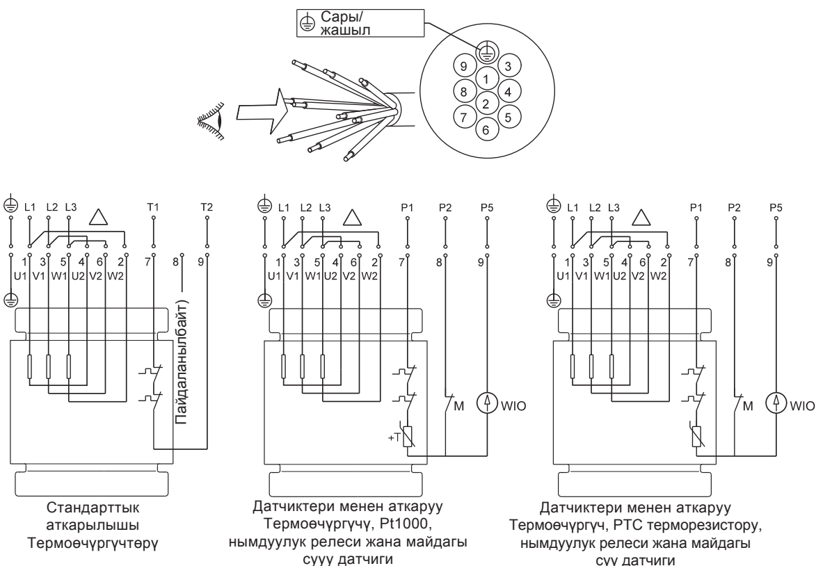
Сүр. 12 10-катмарлуу кабели үчүн электр туташуулардын түзмөктөрү, "үч бурчтук" туташуу (D)
