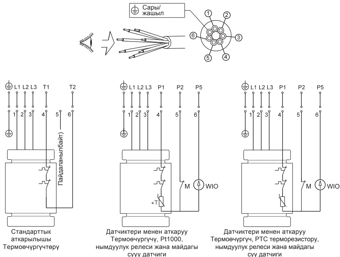
Сүр. 9 7-катмарлуу кабели үчүн электр туташуулардын түзмөктөрү, түз иштетүү
