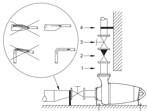
6-сур. Көлденең күйіндегі тіреулердегі құрғақ орнатылым
