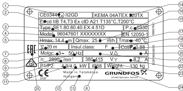
Сүр. 2 Фирмалык тактасы
