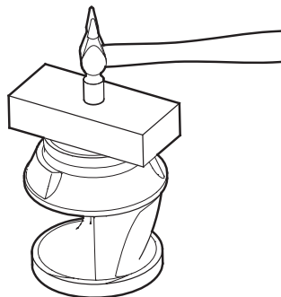
Сүр. 27 Тешиктүү тыгыздооч жээкти орнотуу
