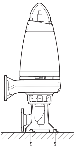
Сүр. 7 Тик негизге кургак орнотуу
