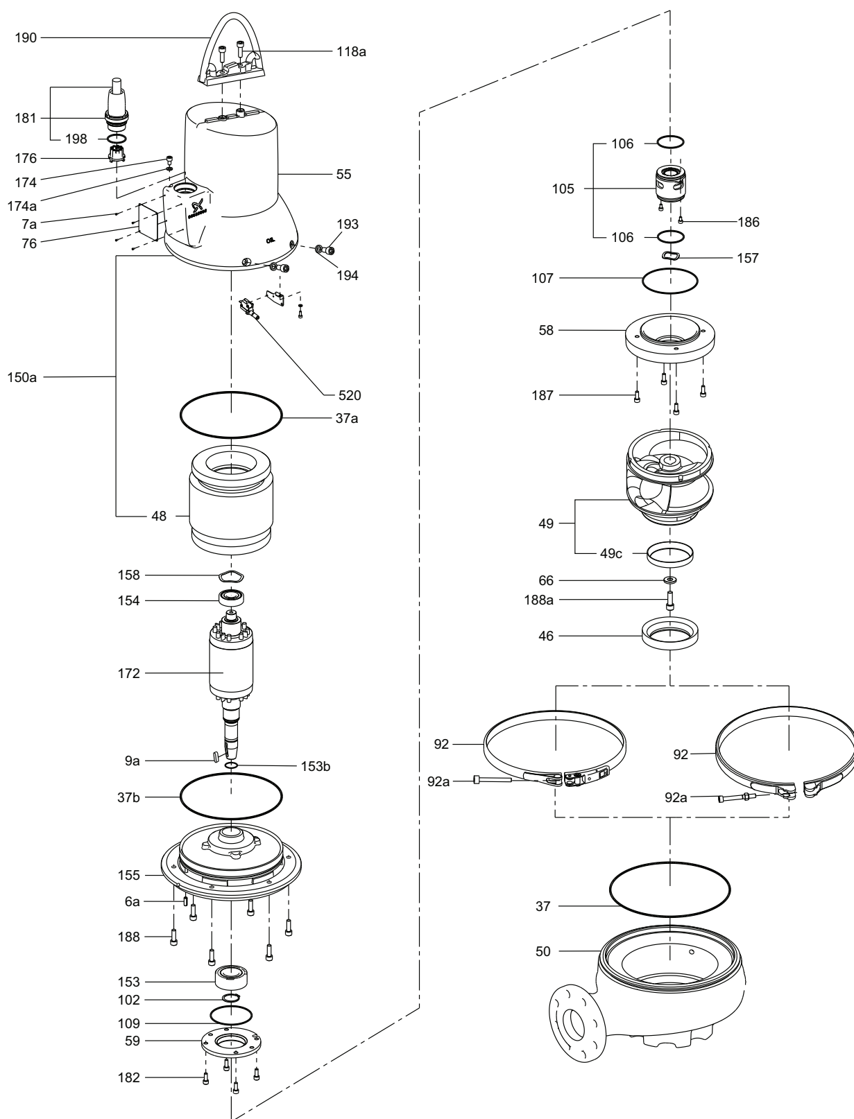
Рис. 8 Детализировка насоса SL1, стандартное исполнение
