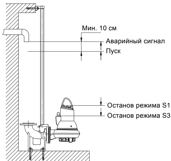
Рис. 14 Уровни пуска и останова насоса
