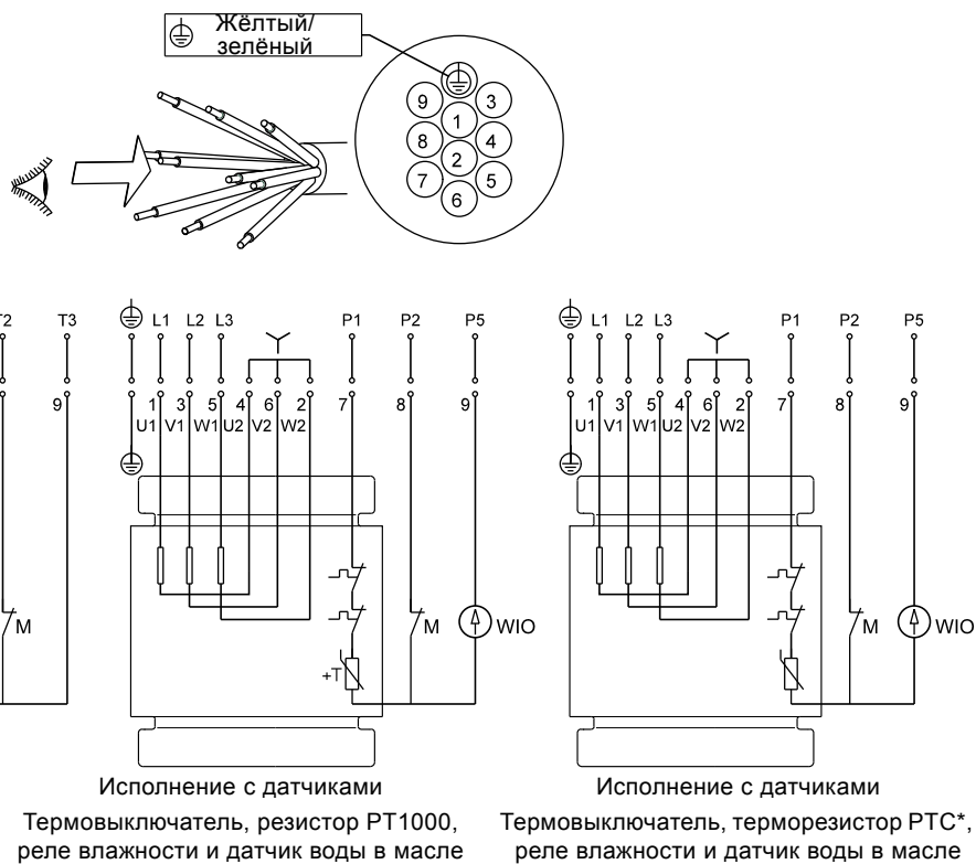
Рис. 8 Схема электрических соединений для 10-жильного кабеля, соединение звездой (Y)
