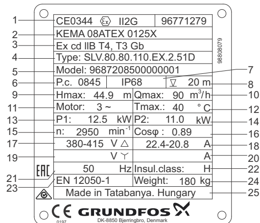
Рис. 3 Фирменная табличка
