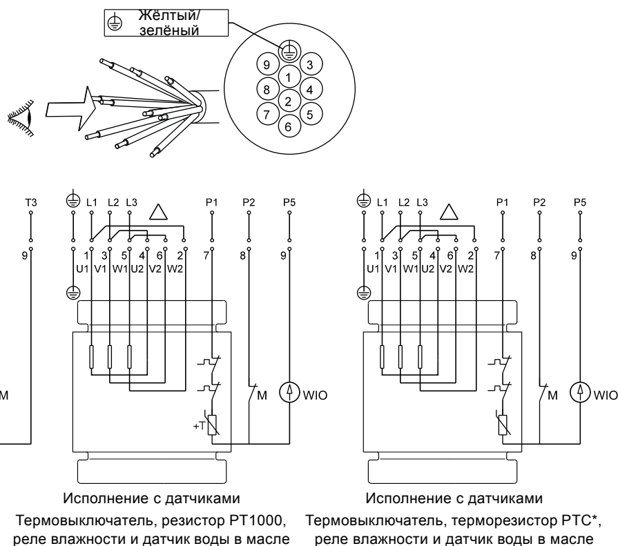
Рис. 9 Схема электрических соединений для 10-жильного кабеля, соединение треугольником (D)
