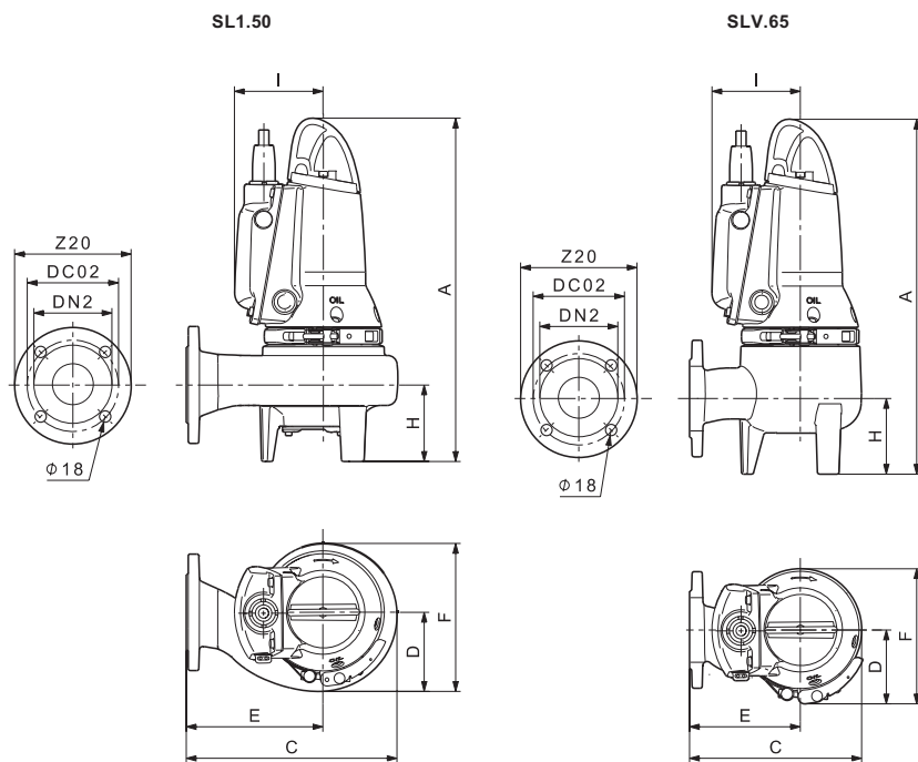
Рис. 20 Свободная установка
