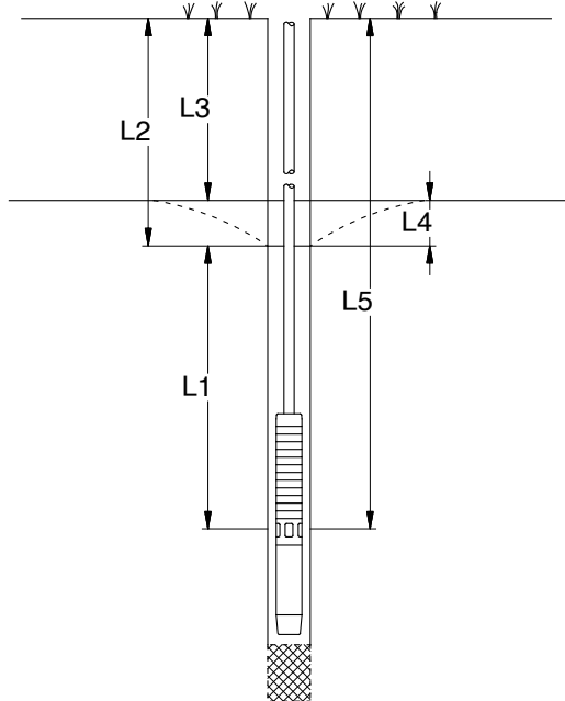
Рис. 28 Сравнение различных уровней воды L1: Минимальная монтажная глубина относительно динамического уровня воды. Рекомендована не менее 1 м. L2: Глубина динамического уровня воды. L3: Глубина статического уровня воды. L4: Снижение уровня. Это разница между динамическим и статическим уровнями воды. L5: Монтажная глубина. Если насос при своей максимальной производительности способен подать объем воды больший, чем способна выработать скважина, рекомендуется установить блок защиты электродвигателя MP 204 производства Grundfos или устройство иного типа для защиты от «сухого» хода. Если защиту от работы насоса «всухую» не устанавливать, то уровень воды может опуститься до той части насоса, в которой находится его всасывающая полость и, как следствие этого, насос начнет подсасывать воздух.
