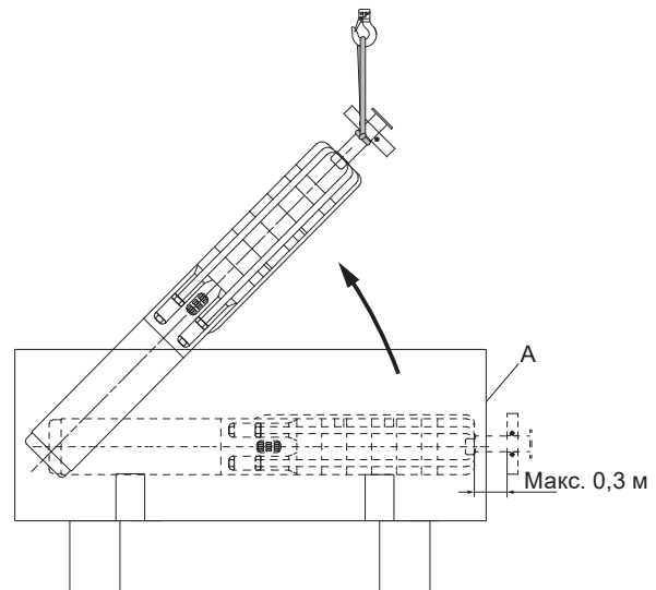
Рис. 12 Подъем и установка насоса в вертикальное положение
