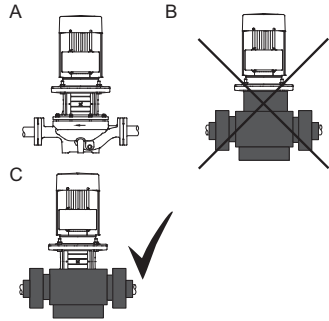
Նկար 18 TP պոմպերի մեկուսացում
