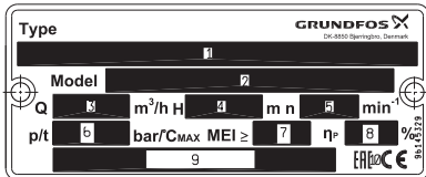
4-сүр. TP, TPD, TPE, TPED соргучтарынын фирмалык табличкасынын үлгүсү
