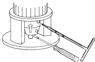
Рис. 20 Затягивание винтов
