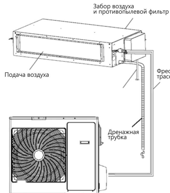
Внутренний блок (типоразмер 18/24/36)
