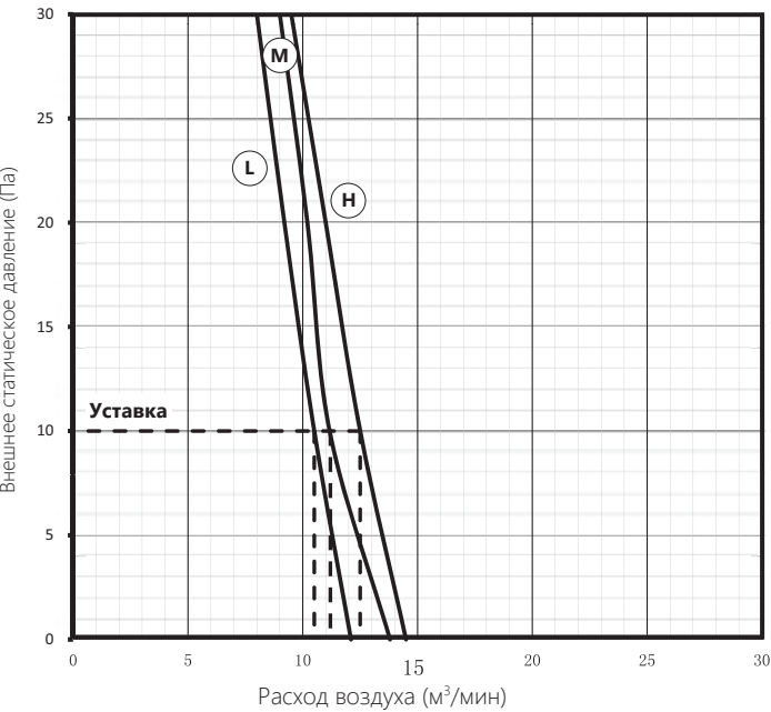
AUD-18HX4SNL1 (уставка 10 Па)
