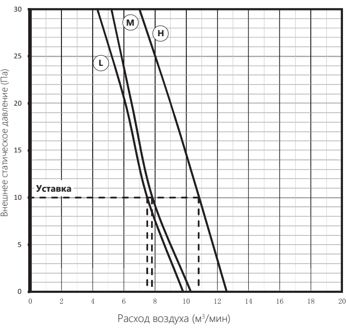
AUD-12HX4SNL (уставка 10 Па)
