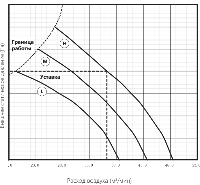
AUD-48HX4SHH (уставка 80 Па)
