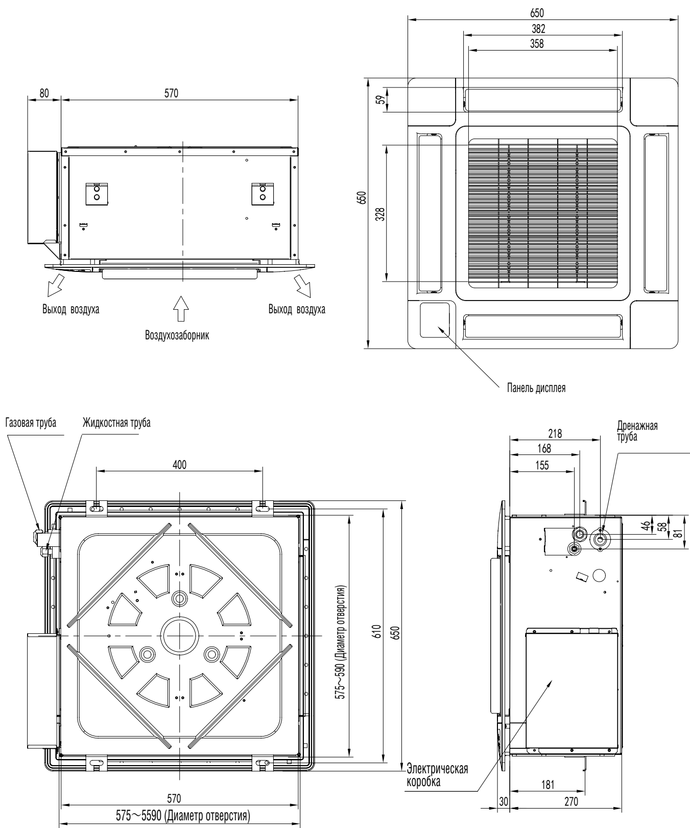
Блоки кассетного типа, типоразмеры 12/18
