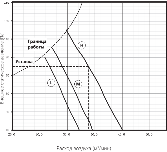
AUD-60HX4SHN (установка 80 Па)
