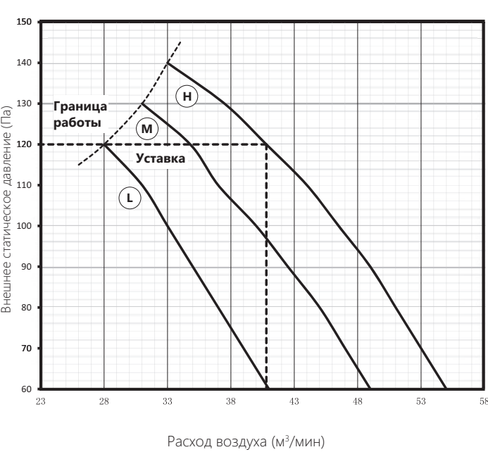
AUD-48HX4SHH (уставка 120 Па)
