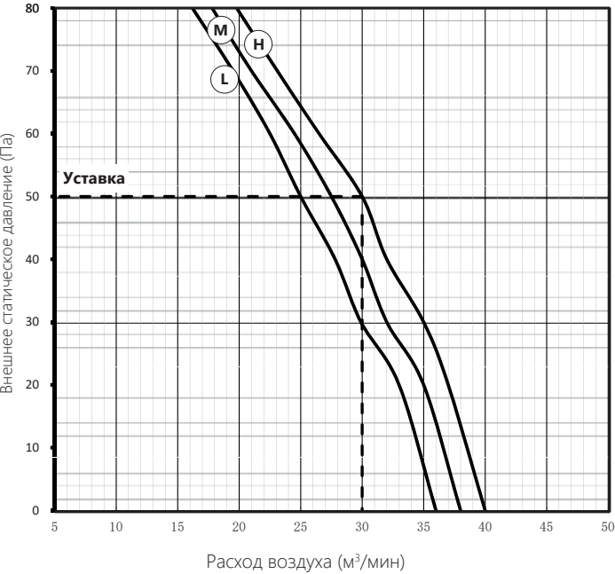
AUD-36HX4SHH1 (уставка 50 Па)
