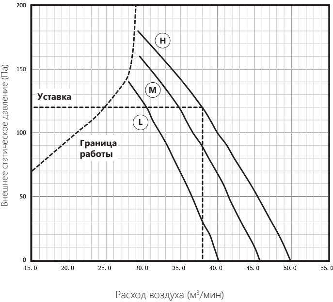
AUD-60HX4SHN (установка 120 Па)
