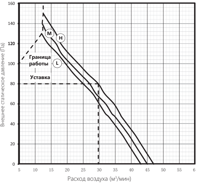
AUD-36HX4SHH1 (уставка 80 Па)
