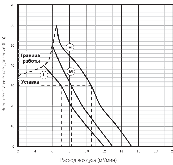
AUD-12HX4SNL (уставка 30 Па)
