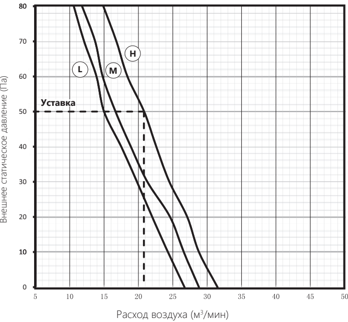
AUD-24HX4SLH1 (уставка 50 Па)
