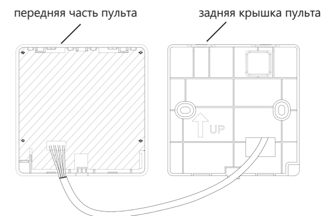
Соединительный кабель
