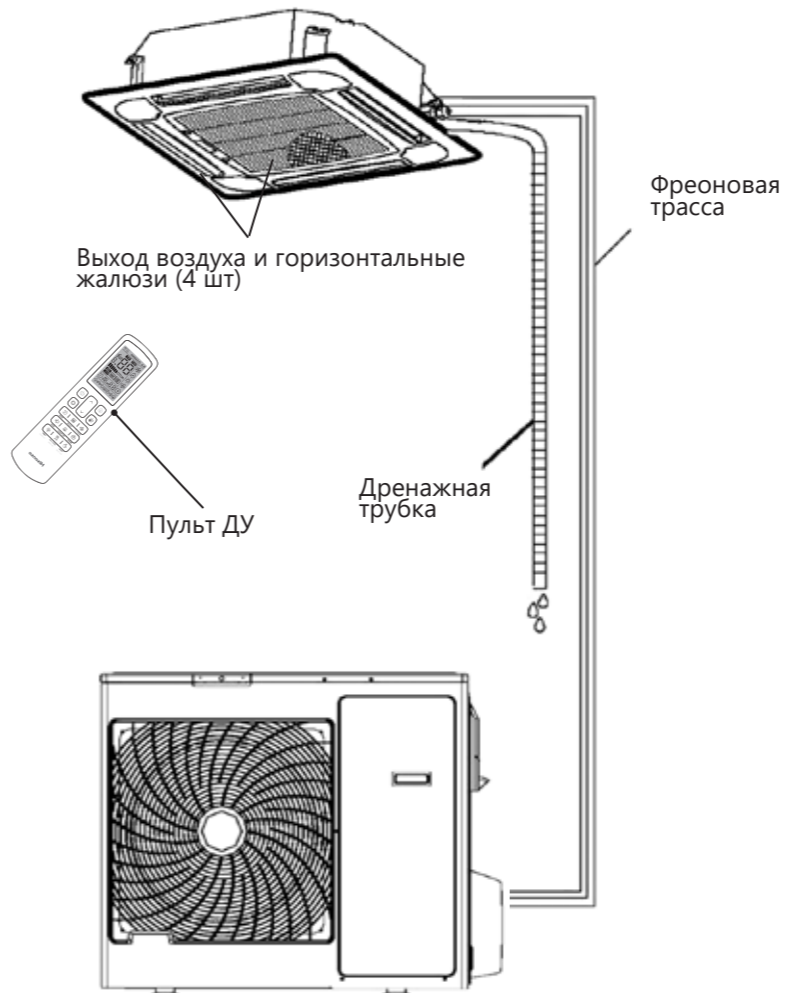
Наружный блок (типоразмер 12/18/24/36/60)
