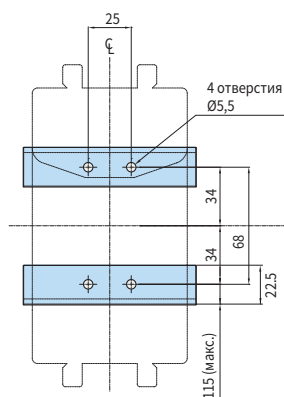
Монтажный чертеж
