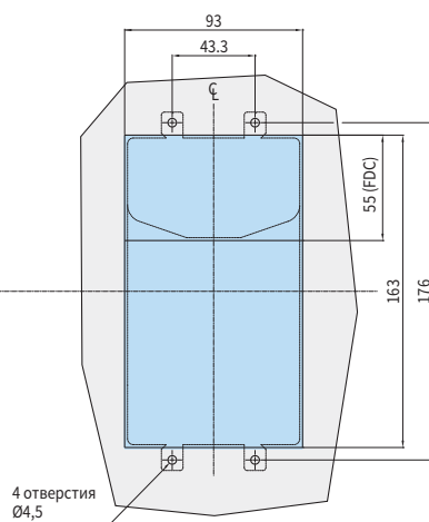
Размеры прорези в передней панели
