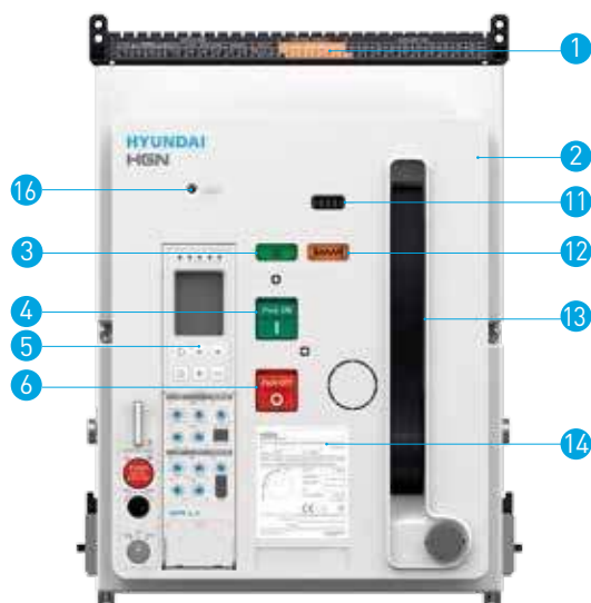
Стационарный тип
