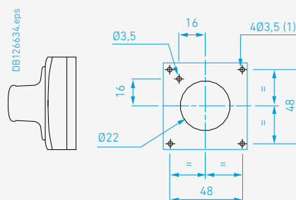
Прорезь на двери
