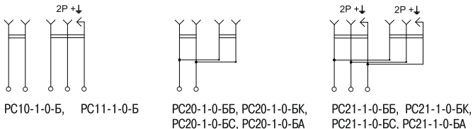
Рисунок 1 – Электрические схемы розеток серии BOLERO
