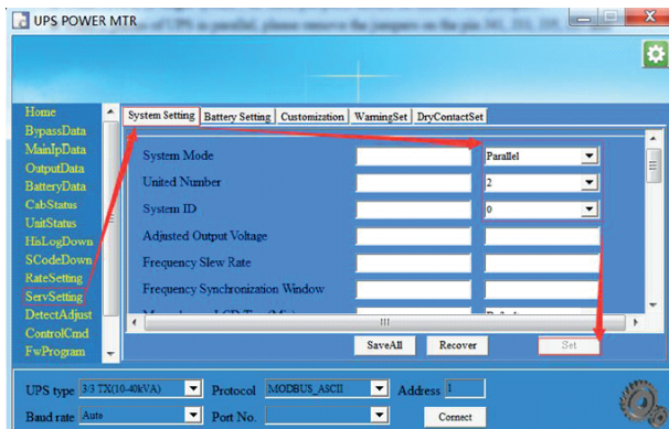
Рисунок 51 – Программа MTR
