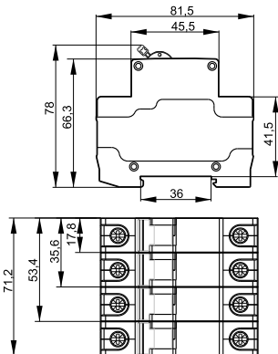
Рисунок 4 – Основные размеры
