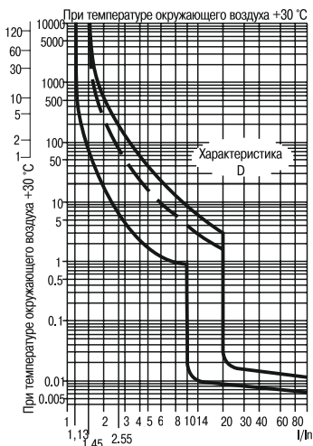
Рисунок 2 – Характеристика D
