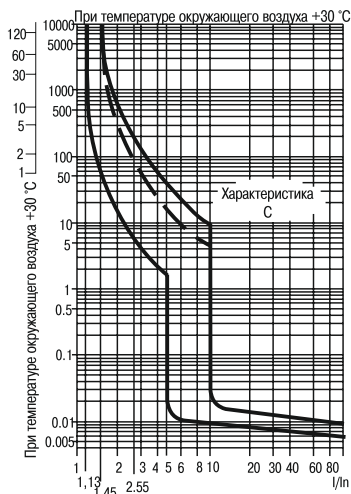
Рисунок 1 – Характеристика C
