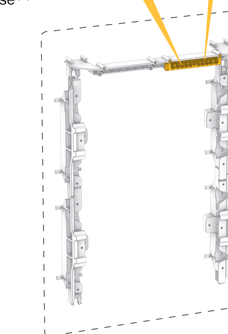
1.5 Установка шин Busbars installation
