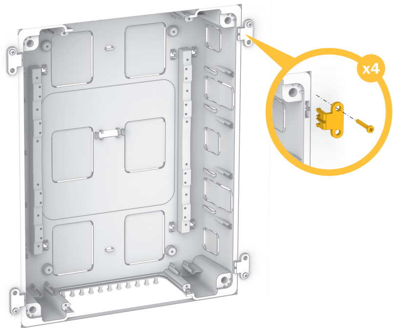
2.2 Крепление в полые стены ЩРВ-П Hollow wall mount
