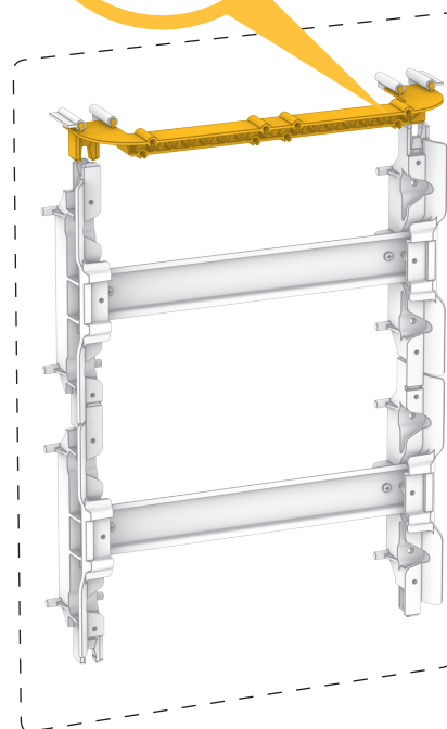
1.4 Крепление кронштейна к основанию** Bracket mount to the base**
