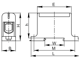
Рисунок 2 – KBC 16-95 (/2), KBC 35-150
