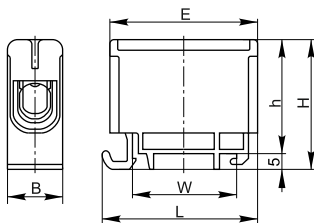
Рисунок 1 – KBC 6-50 (/2, /3)
