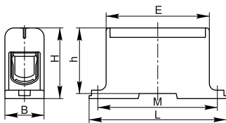
Рисунок 3 – KBC 35-240
