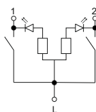
i) выключатель двухклавишный с индикацией / 2-gang switch with indication / индикациясы бар екі пернелі ажыратқыш / întrerupator dublu cu indicatie
