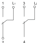
e) выключатель двухклавишный проходной / pass-through 2-gang switch / екі пернелі өтпелі ажыратқыш / întrerupator dublu de trecere prin
