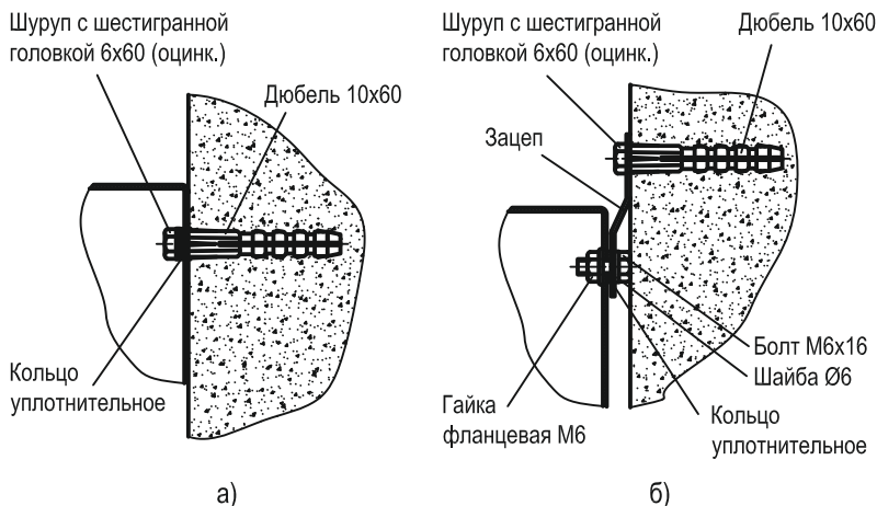
Рисунок 3 – Крепление металлокорпуса к стене
