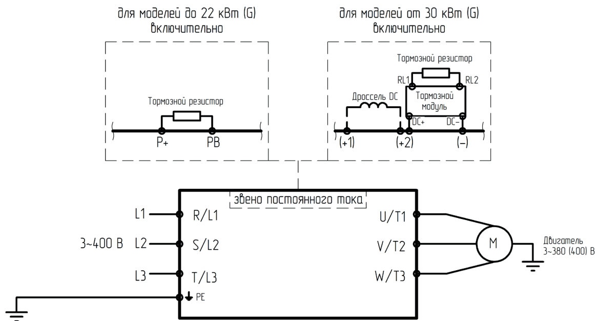
Рисунок 3. Подключение силовых клемм
