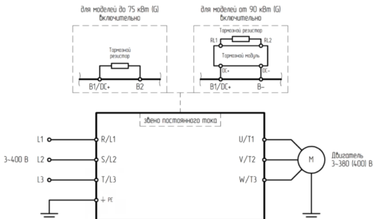
Рис. 3.2 - Схема силовых подключений для серии INPRIME
