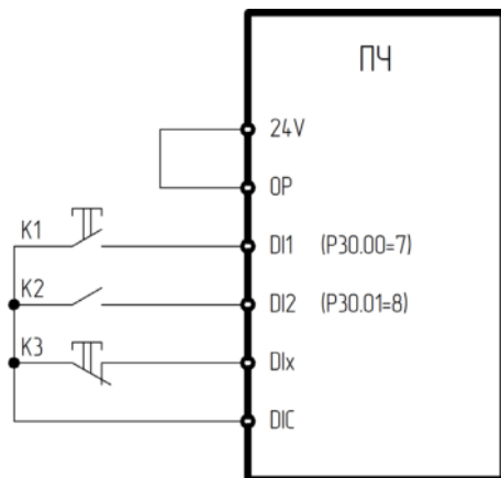
Рис. 6.4 - Трехпроводной режим работы 2
