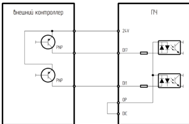
Рис.3.11 - Режим подключения внутреннего питания +24 В с логикой PNP
