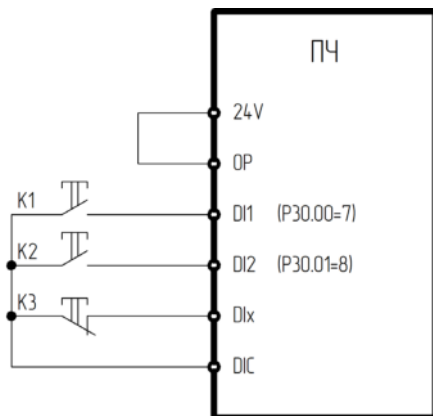
Рис. 6.3 - Трехпроводной режим 1
