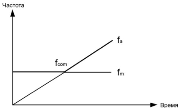
Рис. 6.25 - Комбинация «Максимальное значение» каналы задания частоты
