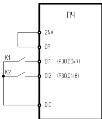
Рис. 6.1 - Двухпроводной режим 1
