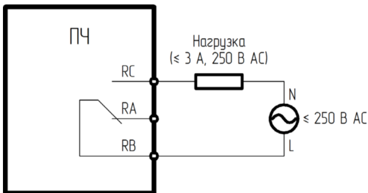
Рис. 3.15 - Схема подключения нагрузки переменного тока к релейному выходу
