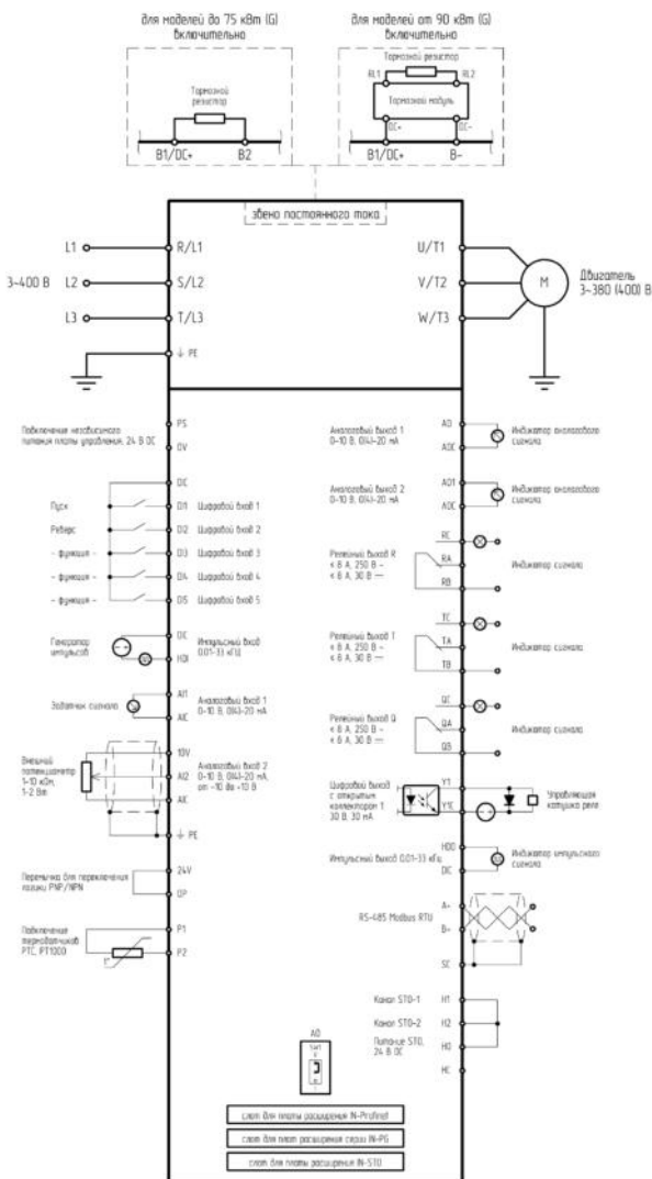
Рис. 3.46 - Схема подключения управляющих клемм серии INPRIME (плата IN-I/O-B)
