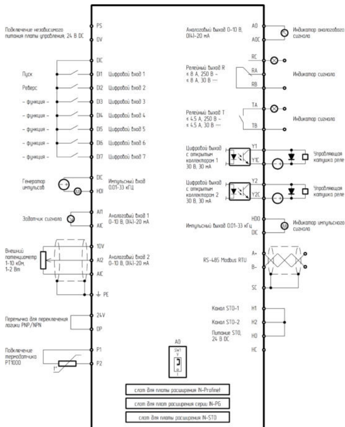
Рис. 3.4а - Схема подключения управляющих клемм серии INPRIME (плата IN-I/O-A)
