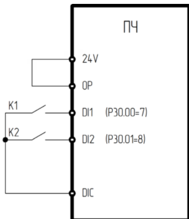
Рис. 6.2 - Двухпроводной режим 2
