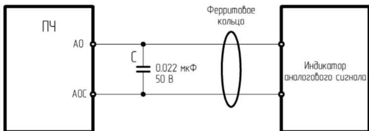
Рис. 3.17 - Схема подключения индикатора аналогового сигнала к аналоговому выходу
