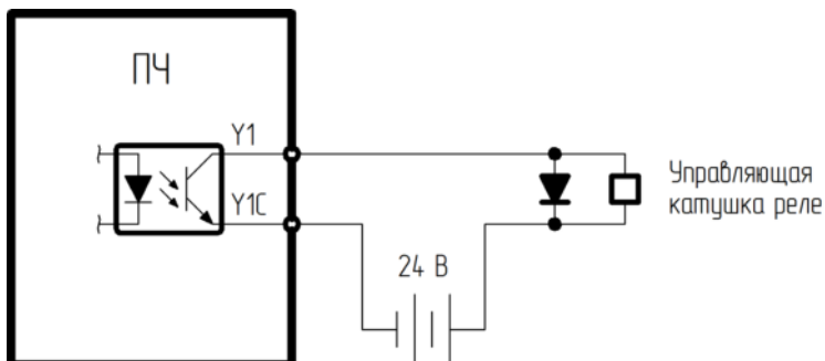
Рис. 3.14 - Схема подключения цифрового выхода с открытым коллектором.
