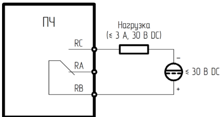
Рис. 3.16 - Схема подключения нагрузки постоянного тока к релейному выходу
