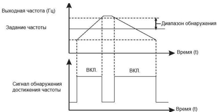
Рис. 6.17 Диапазон достижения максимальной частоты
