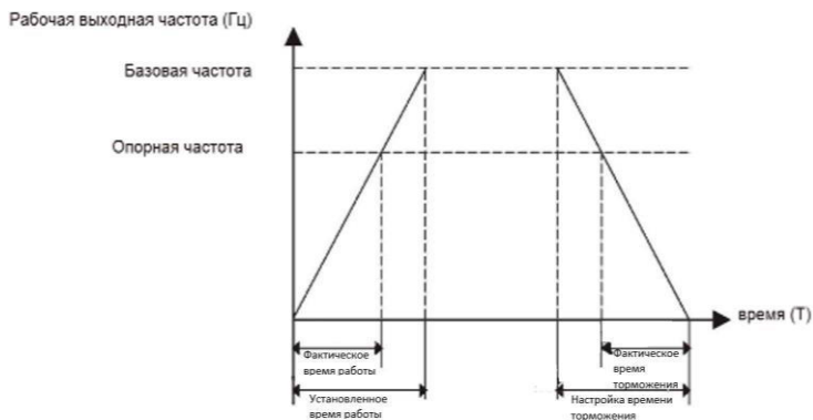
Рис. 6.1 Время разгона/торможения
