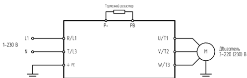
Рис. 3.2.2 Подключение силовых клемм
