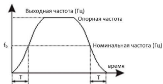
Рис. 6-3 Кривая S разгона/торможения B
