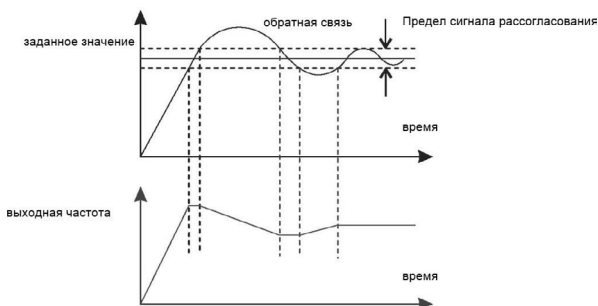
Рис.6.24. Отклонение ПИД-управления
