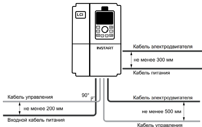
Рис. 3.6 Графическое представление расстояний между кабелями
