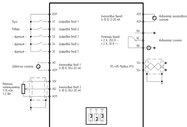
Рис. 3.4а Схема подключения управляющих клемм серии LCI(S)
