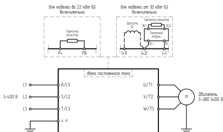
Рис. 3.2.4 Подключение силовых клемм
