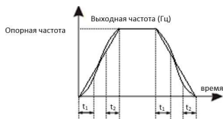
Рис. 6-2 Кривая S разгона/торможения A
