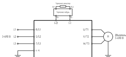
Рис. 3.2.5 Подключение силовых клемм
