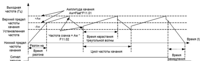
Рис. 6.27. Иллюстрация функции частоты качания
