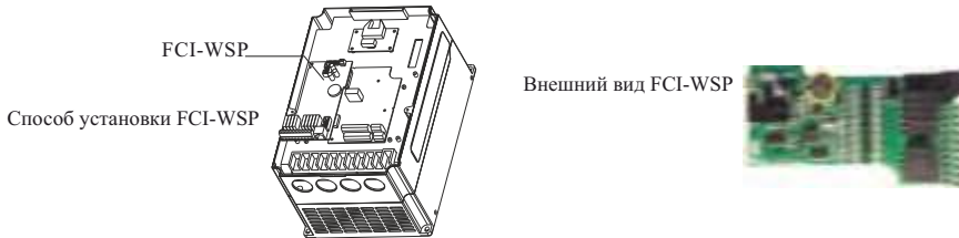
Клеммы FCI-WSP
