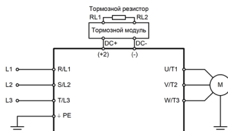
Рис. 3.2.5 Подключение силовых клемм
