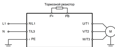
Рис. 3.2.2 Подключение силовых клемм
