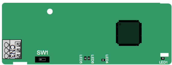
A.5.4 Коммуникационная плата CANopen (EC-TX505) и коммуникационная плата управления главным/подчиненным устройствами CAN (EC-TX511)
