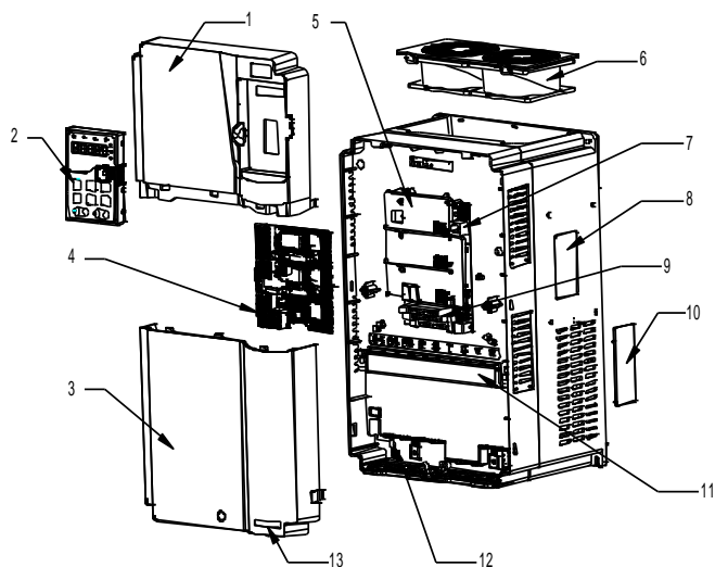
Рисунок 3-7 Конструкционная схема
