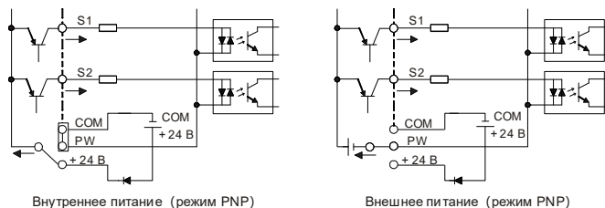
Рисунок 4-21 режим PNP
