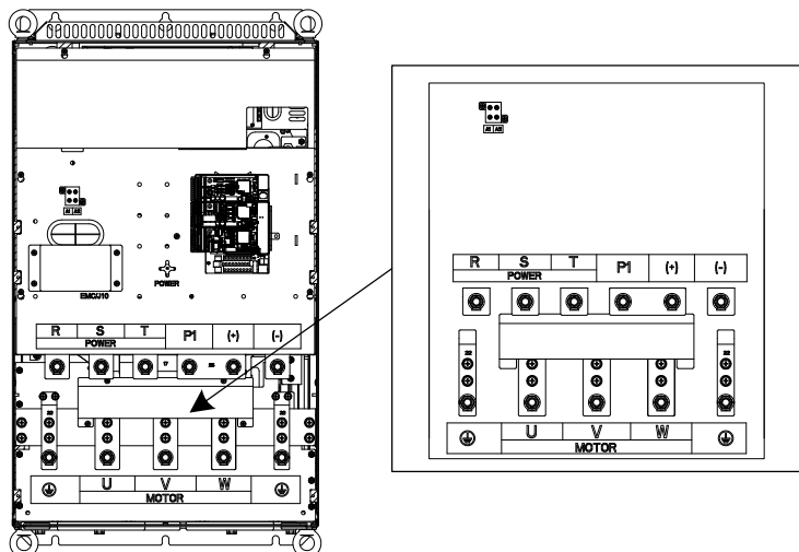
Рисунок 4-14 Схема клемм главной цепи для 380 В 132–200 кВт (без A1 или A2) и 660 В 160–220 кВт
