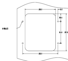
Рисунок С-2 (стандарт) Монтажный кронштейн для моделей 380 В, 37–315 кВт и 660 В, 22–630 кВт
