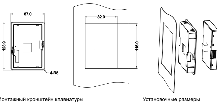
Рисунок C-1 (дополнительно) Монтажный кронштейн для моделей 380 В, 1,5–315 кВт и 660 В, 22–630 кВт
