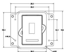
Монтажный кронштейн клавиатуры
