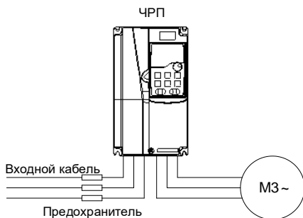
Рисунок 4-24 Конфигурация предохранителя
