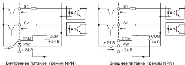
Рисунок 4-20 Режим NPN
