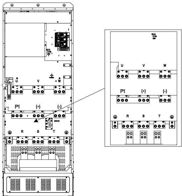
Рисунок 4-16 Схема клемм главной цепи для 380 В 355–500 кВт (без А1 или А2) и 660 В 400–630 кВт
