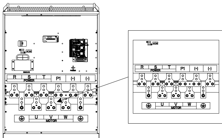
Рисунок 4-15 Схема клемм главной цепи для 380 В 220–315 кВт (без A1 или A2) и 660 В 250–355 кВт
