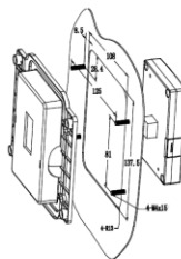
Установочные размеры
