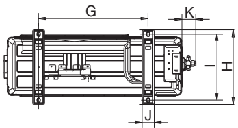
Наружный блок
