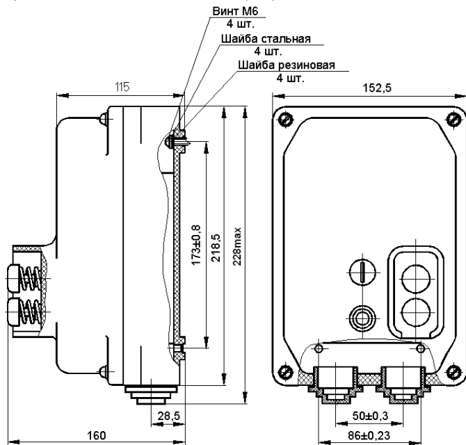
Рисунок В.3 – Выключатель в дополнительной оболочке (двух- и трехполюсный)
