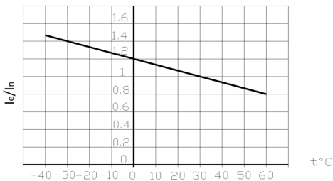
Рисунок Г.4 – Зависимость номинального рабочего тока выключателей от температуры окружающего воздуха
