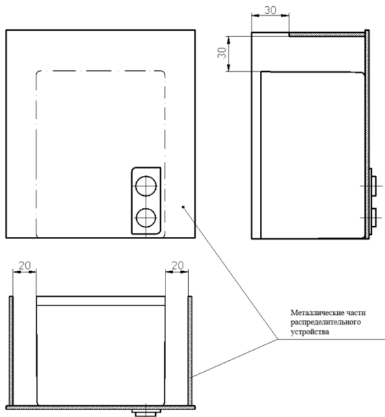
Рисунок Д.1 – Минимальные допустимые расстояния между металлическими частями распределительного устройства и выключателем
