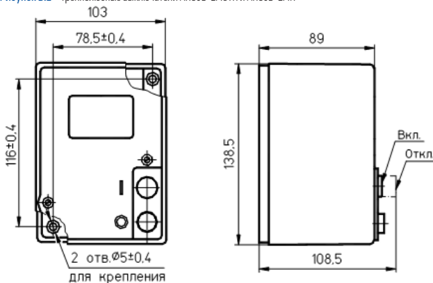
Рисунок В.2 – Трехполюсные выключатели АП50Б-2МЗТН и АП50Б-2МН
