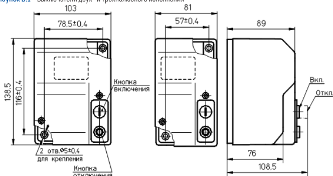
Рисунок В.1 – Выключатели двух- и трехполюсного исполнения
