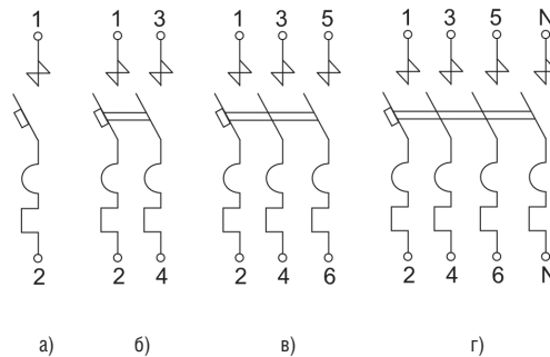
Рисунок Г.1 а) однополюсного; б) двухполюсного с двумя защищенными полюсами; в) трехполюсного с тремя защищенными полюсами; г) четырехполюсного с четырьмя защищенными полюсами.
