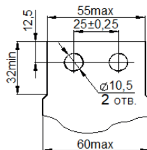
Рисунок Д.2 – Форма и размеры присоединяемой шины максимального сечения
