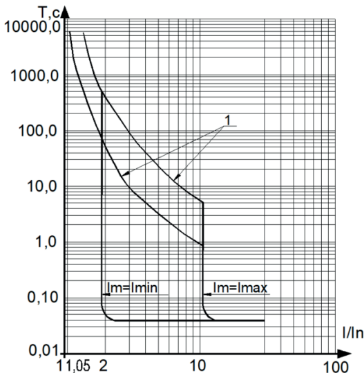
Рисунок А.1 – Время-токовые характеристики (справочные) выключателей при одновременной нагрузке всех полюсов с холодного состояния при контрольной температуре
