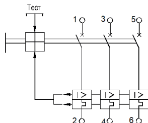
Рисунок В.2 – Выключатель двухполюсного исполнения:
