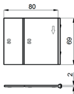
Рисунок Б.5 – Выключатель с выводами для заднего присоединения
