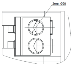
Рисунок Д.2 – Форма и размеры присоединяемой шины максимального сечения
