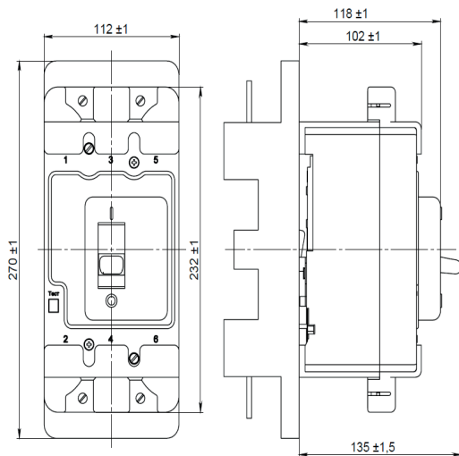
Рисунок Б.11 – Выключатель ВА57-35 с электромагнитным приводом на втычной панели
