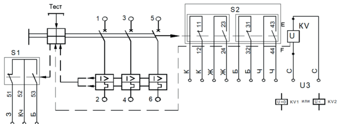
Рисунок Г.4 – Схема электрическая принципиальная выключателей стационарного исполнения, с нулевым или минимальным расцепителем напряжения, вспомогательными контактами сигнализации автоматического отключения, вспомогательными контактами и электромагнитным приводом
