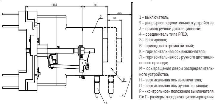
Рисунок Б.8 – Выключатель ВА57-35 выдвигного исполнения с электромагнитным приводом
