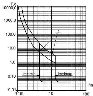
Рисунок А.6 – Время-токовые характеристики выключателей на токи 160, 200, 250 А
