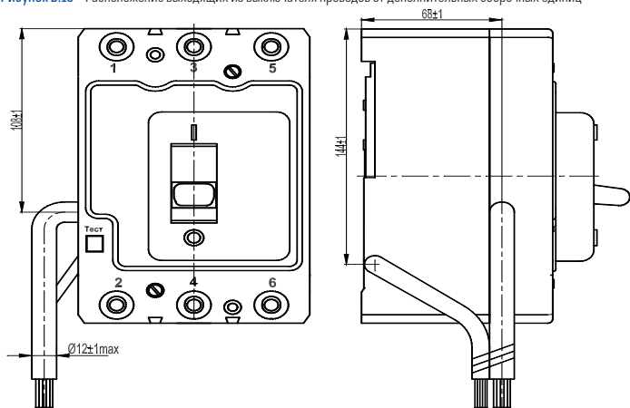
Рисунок Б.13 – Расположение выходящих из выключателя проводов от дополнительных сборочных единиц
