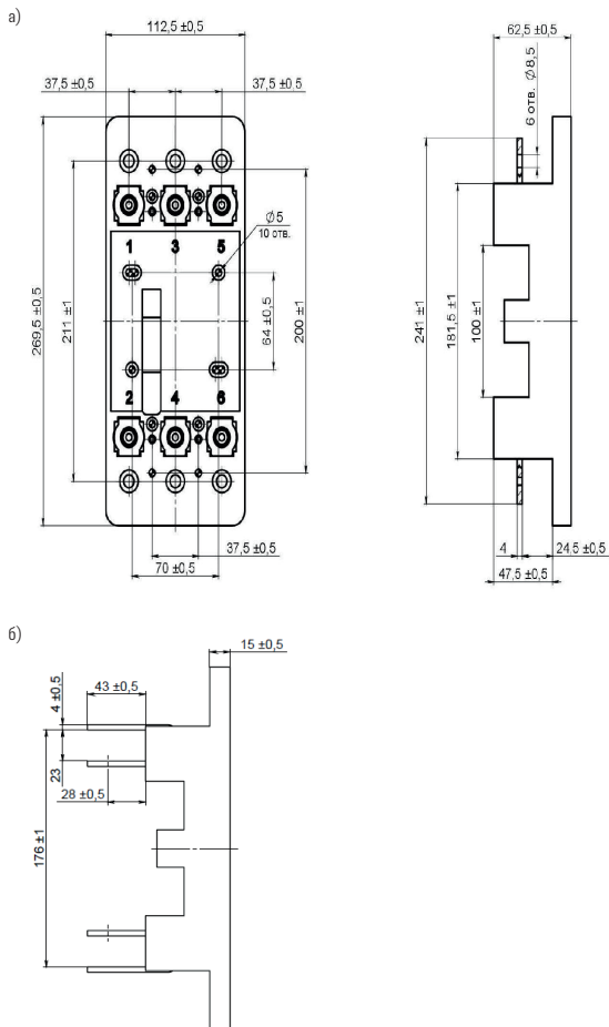
Рисунок 5.9 – Панель втычная ВА57-35
