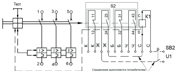
Рисунок Г.3 – Схема электрическая принципиальная выключателей стационарного исполнения, с нулевым или минимальным расцепителем напряжения, вспомогательными контактами сигнализации автоматического отключения и вспомогательными контактами
