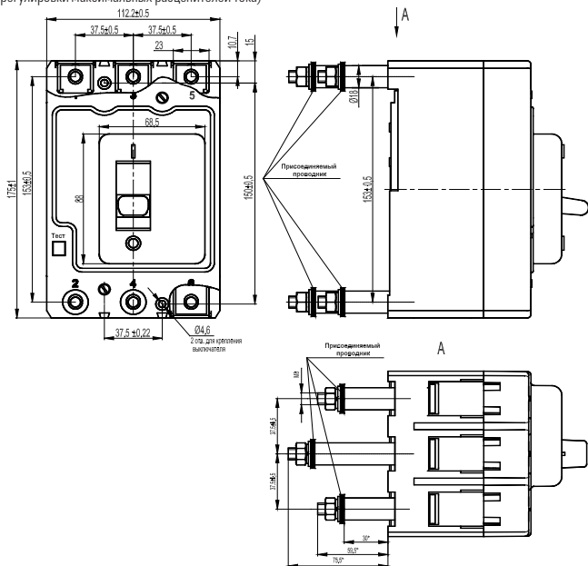
Рисунок 5.2 – Выключатели с зажимами для заднего присоединения (только ВА57-35 стационарного исполнения без регулировки максимальных расцепителей тока)
