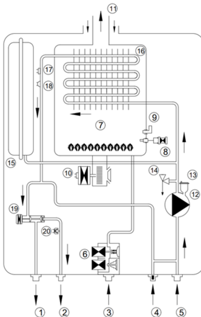
1. Выход теплоносителя в систему отопления («подача») 11. Выход продуктов сгорания/забор воздуха 2. Выход теплоносителя в бойлер ГВС 12. Насос циркуляционный 3. Вход газа 13. Воздухоотводчик 4. Вход теплоносителя из бойлера ГВС 14. Клапан предохранительный 5. Вход теплоносителя («обратка») 15. Расширительный бак 6. Клапан газовый 16. Теплообменник первичный 7. Горелка 17. Датчик перегрева теплообменника 8. Электроды розжига 18. Датчик температуры теплоносителя 9. Датчик пламени (фотоэлемент) 19. Трехходовой клапан 10. Вентилятор 20. Датчик давления теплоносителя
