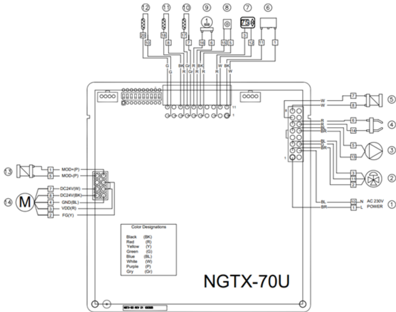
Рисунок 16. Схема электрическая.
