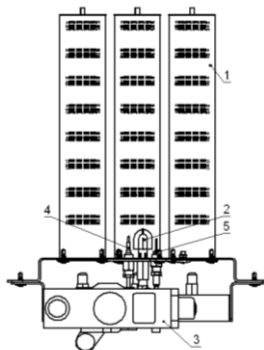
рис.8 Горелки УГ-29S к АОГВ/ АКГВ-23,2-3-2; УГ-33S к АОГВ/ АКГВ-29-3-2
