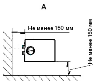
Схема установки аппаратов
