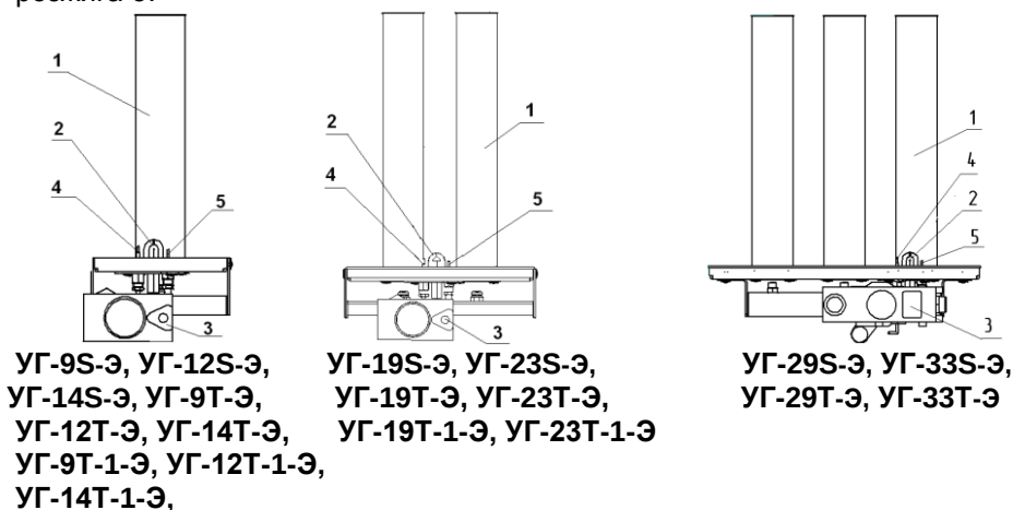
Рис.6 Газогорелочные устройства с автоматикой безопасности и регулирования.
