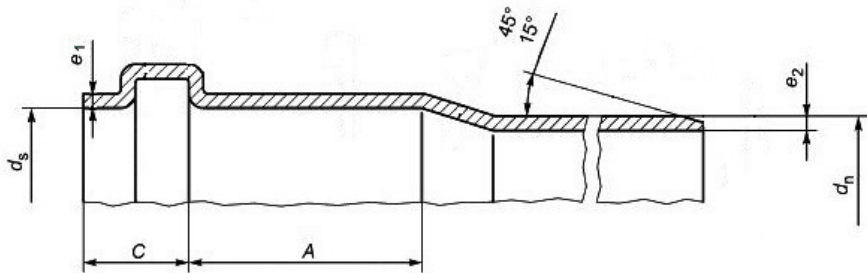
Рисунок 1. Размеры раструбов и трубных концов.
